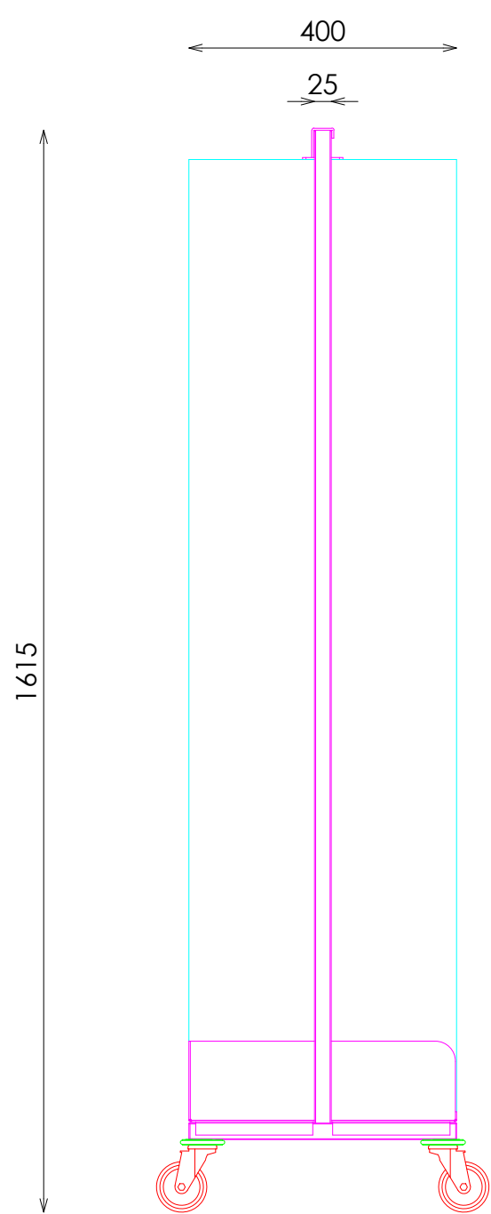
ALZADO LATERAL
