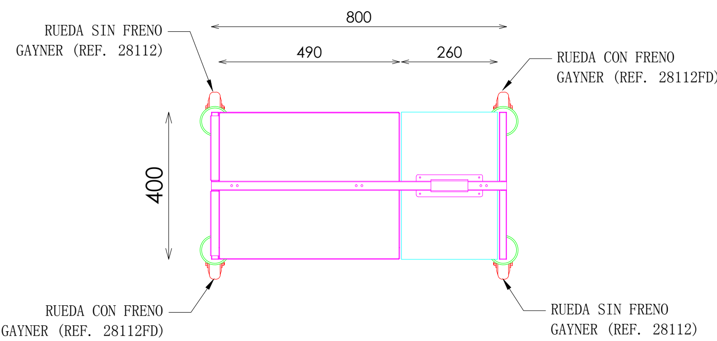
PLANTA
