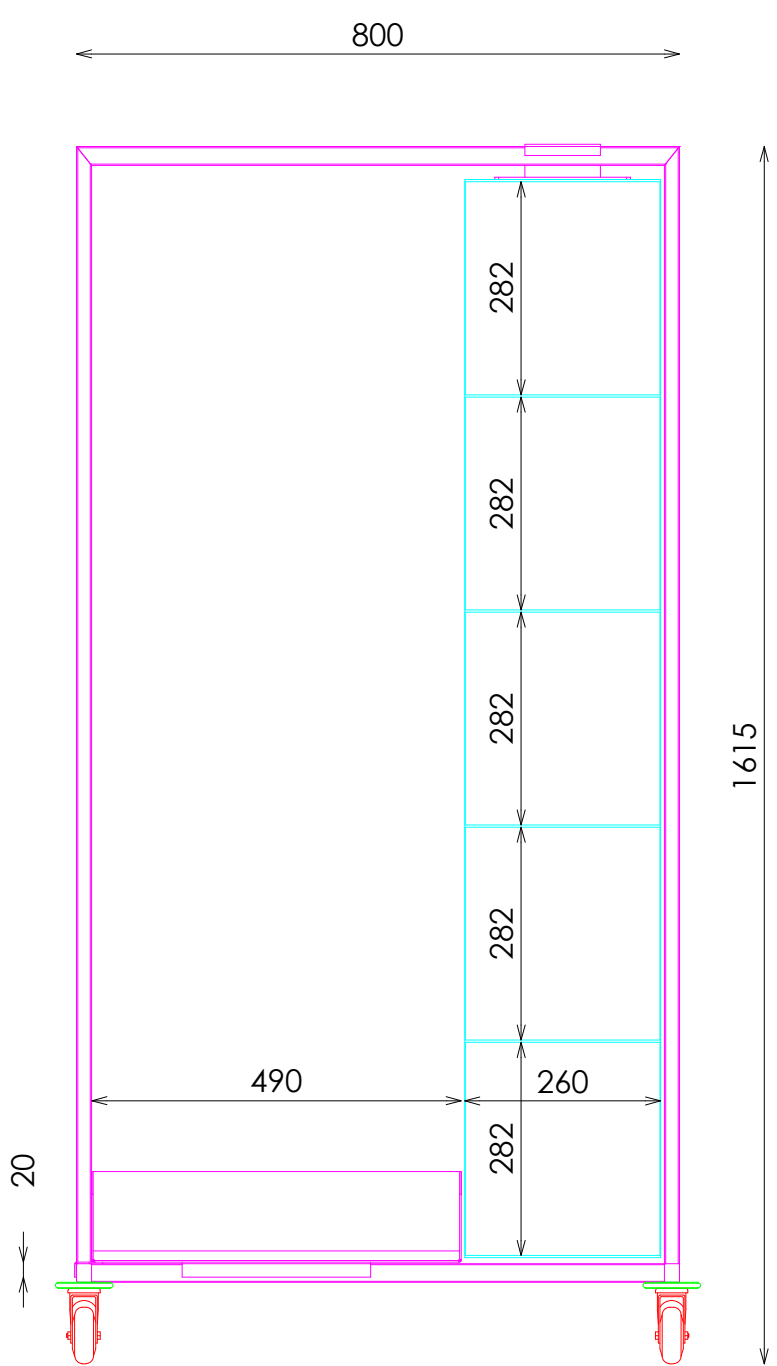
ALZADO FRONTAL
