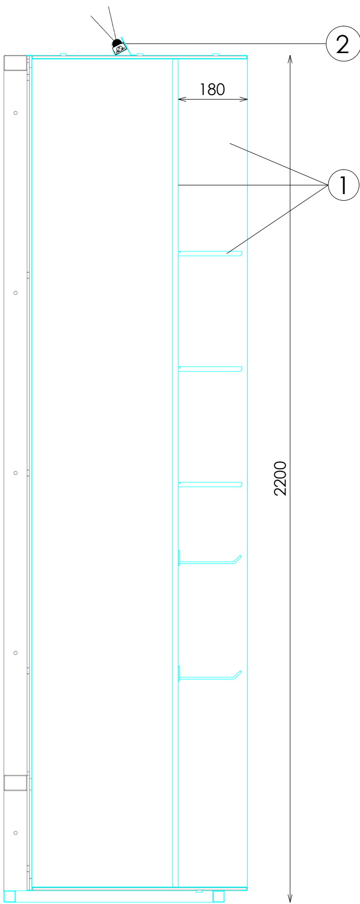
SECCIÓN
