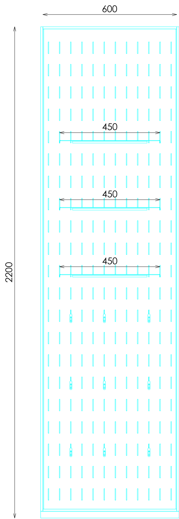
ALZADO
