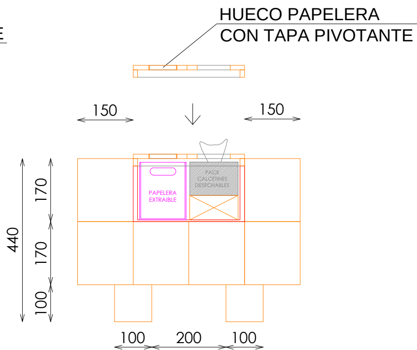
SECCIÓN TRANSVERSAL
