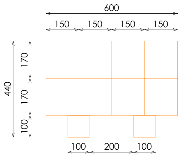
PERFIL
