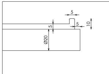
DETALLE C
