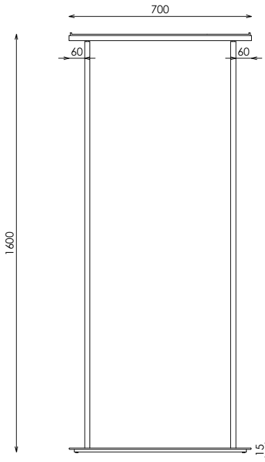
ALZADO
