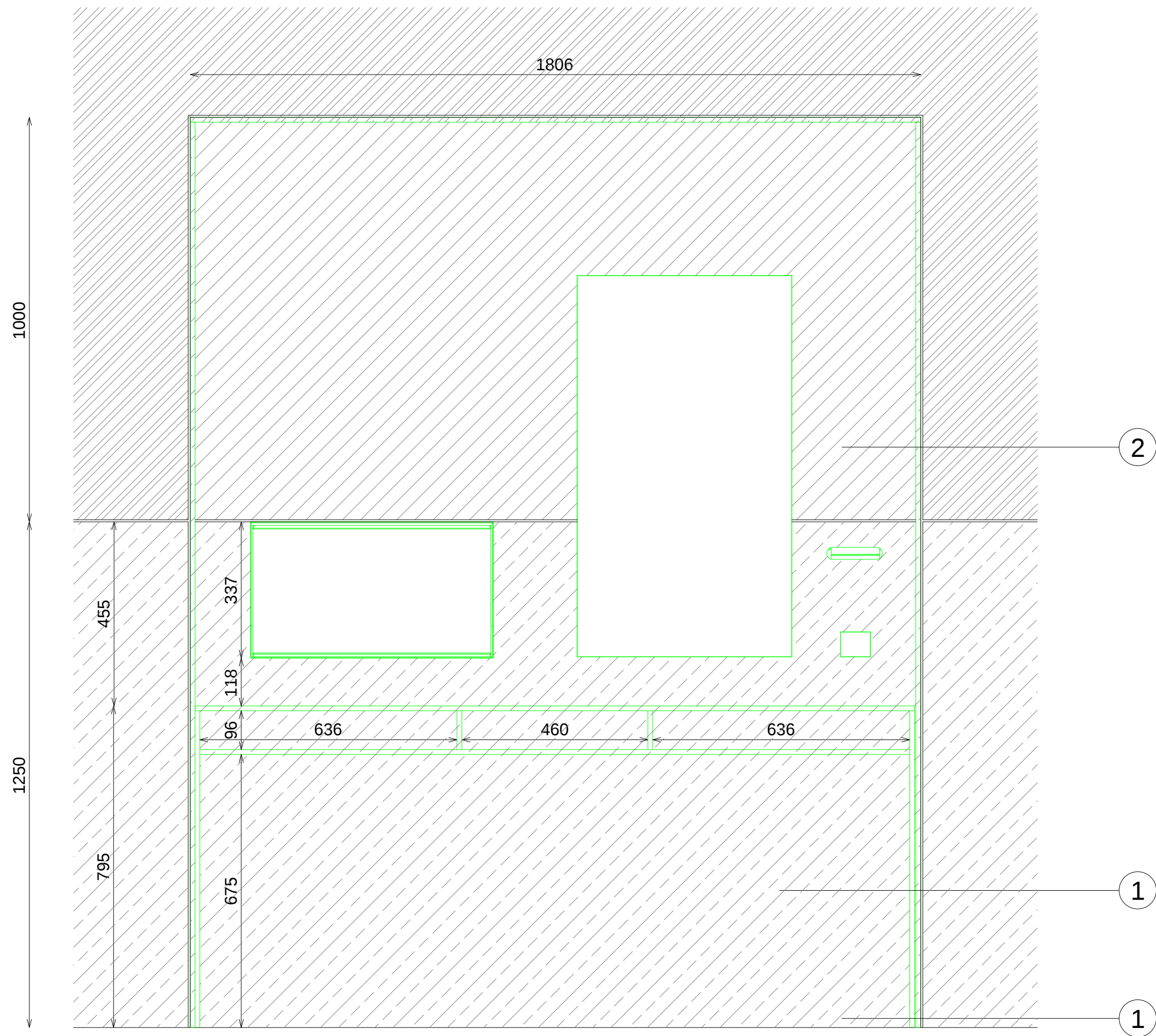
ALZADO FRONTAL
