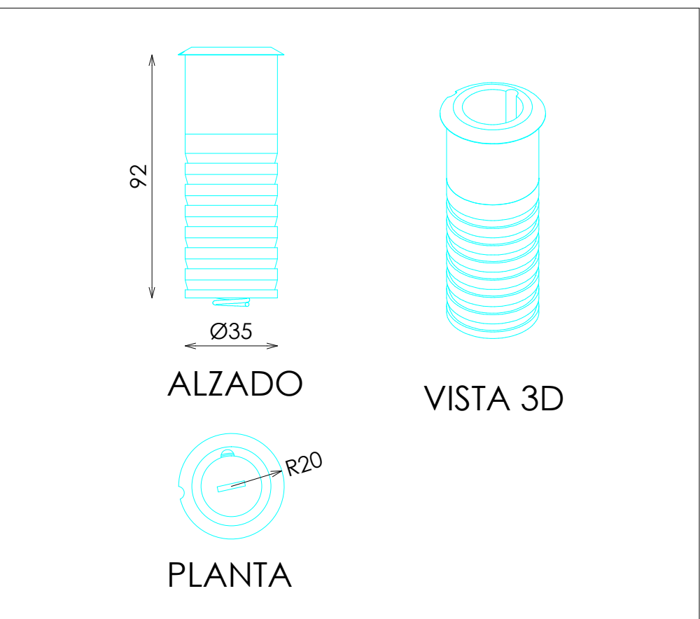
CASQUILLO FIJACIÓN POSTE-SUELO
