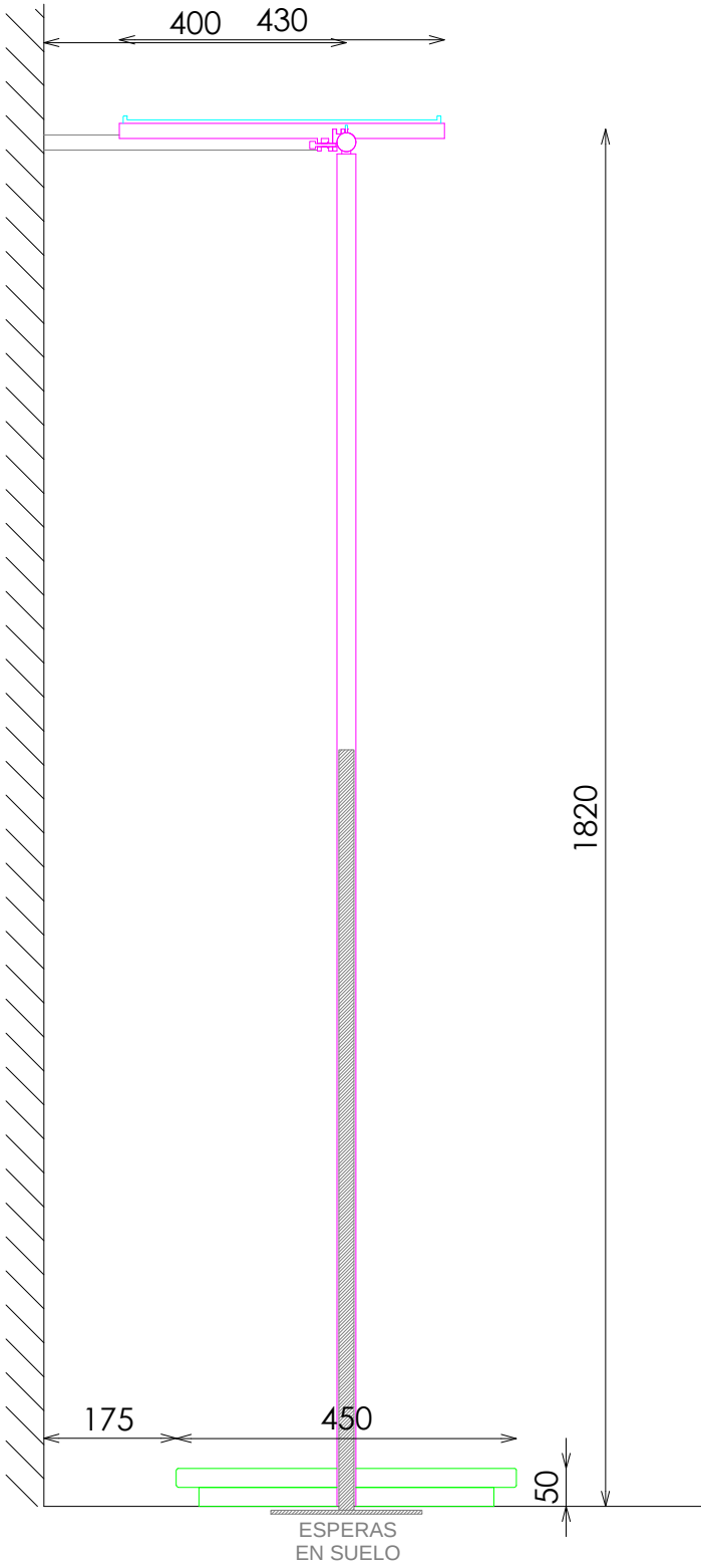
SECCIÓN
