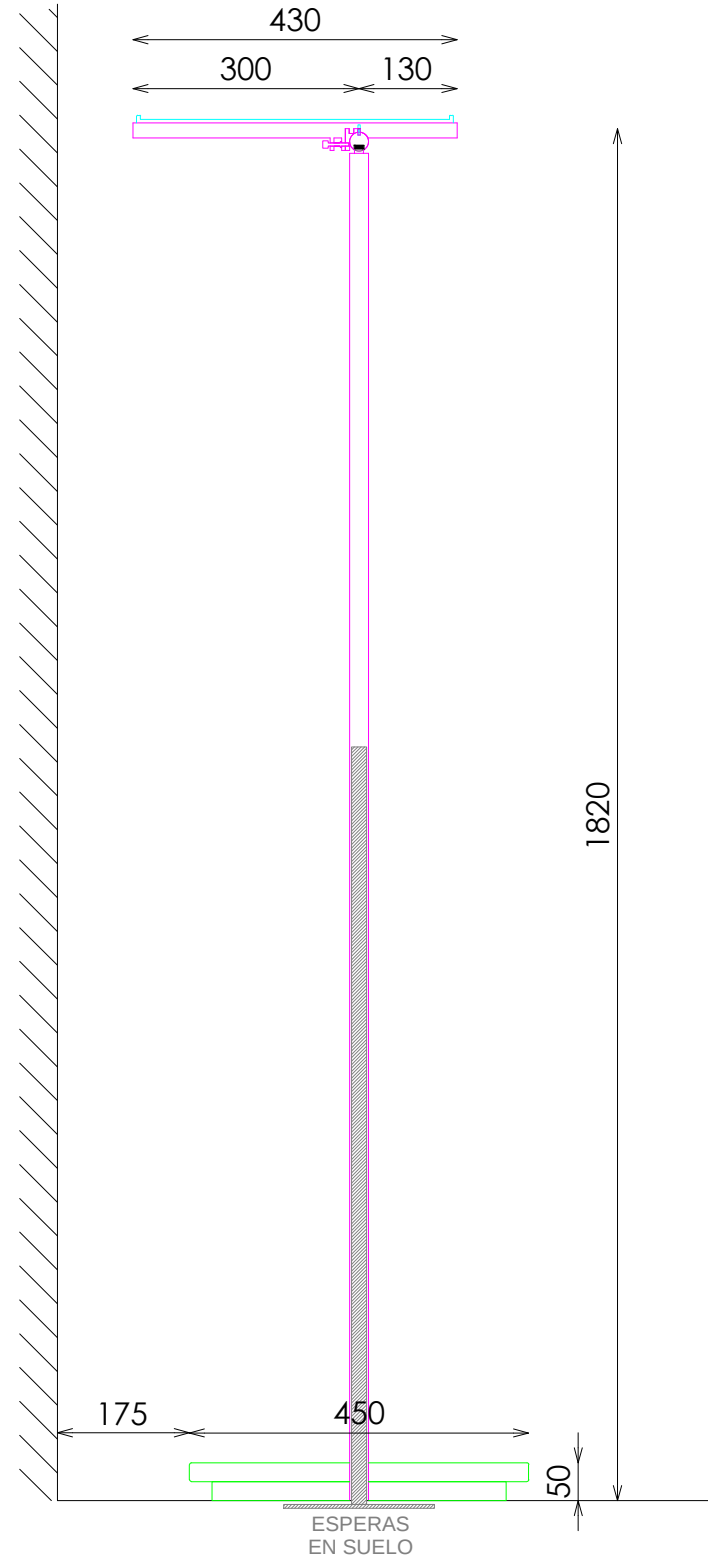
SECCIÓN
