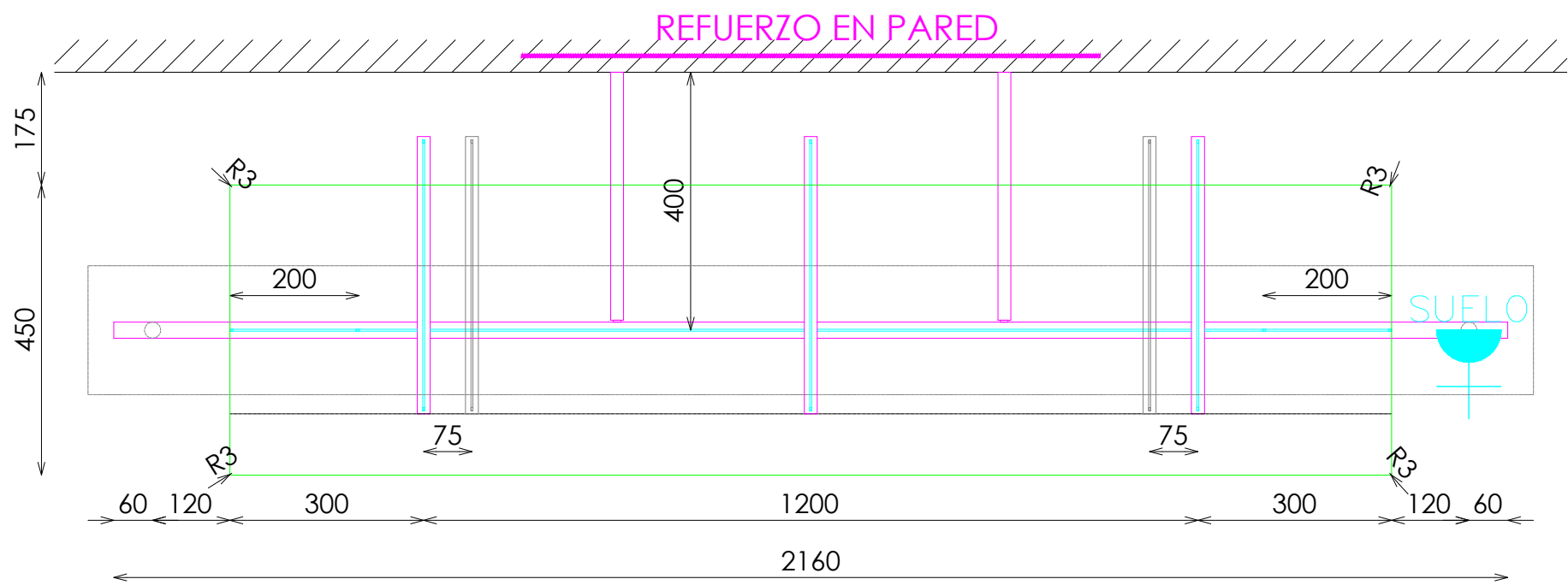
PLANTA
