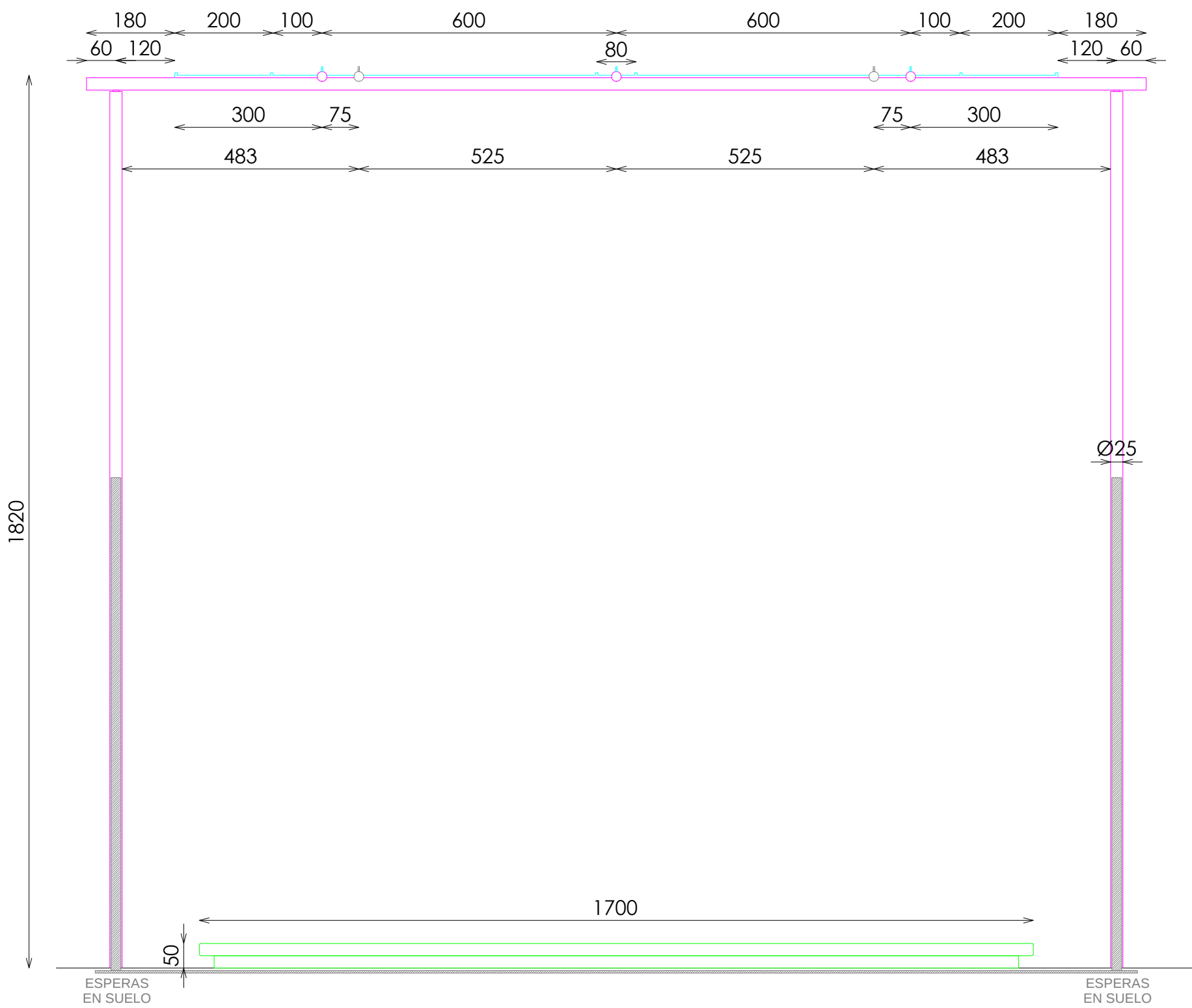
ALZADO FRONTAL
