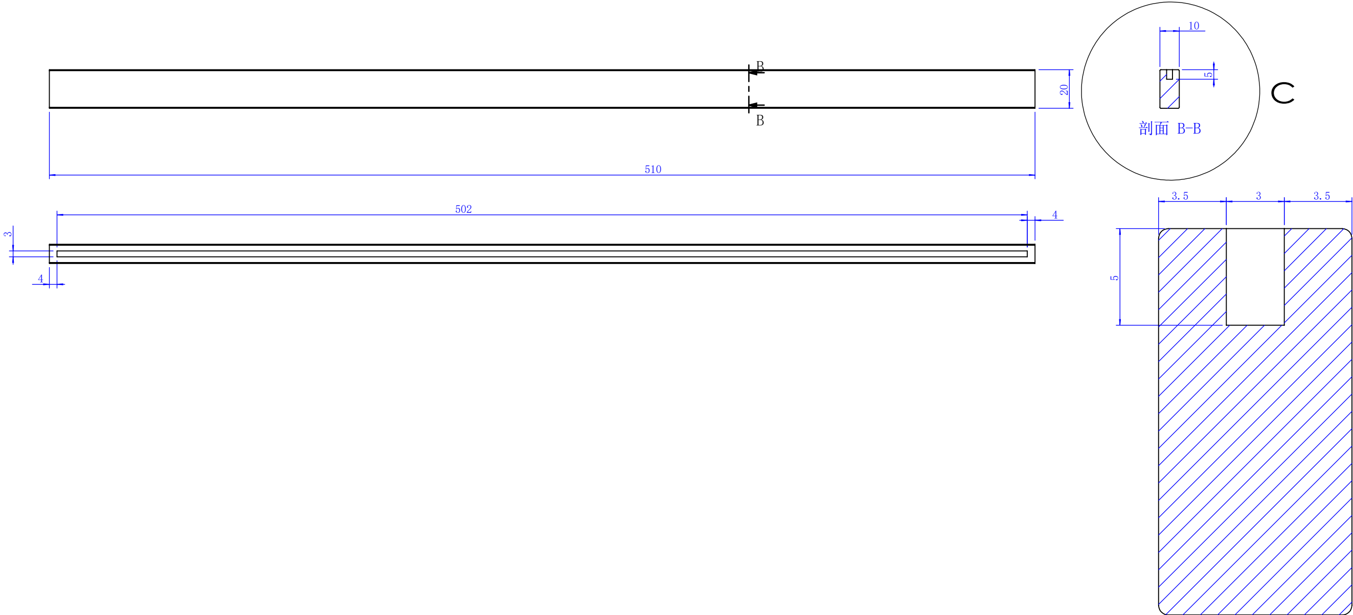
局部视图 C 比例 5 : 1
