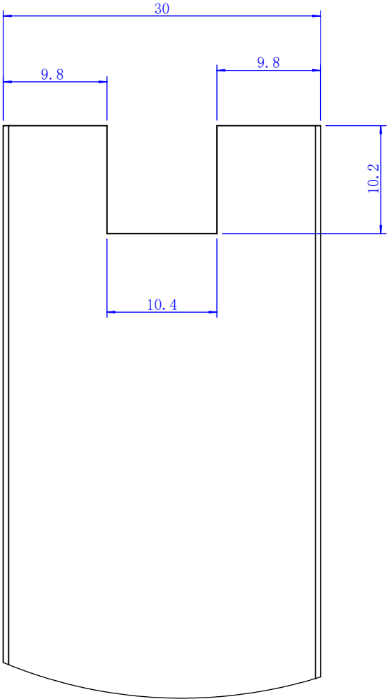
局部视图 D 比例 2 : 1
