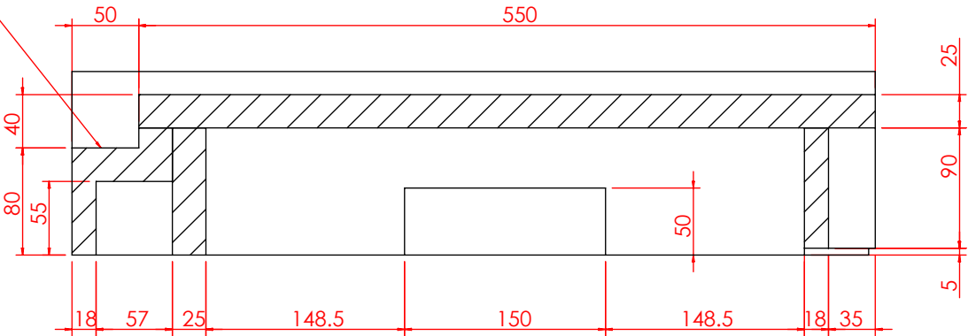
局部视图 AH 比例 1 : 5
