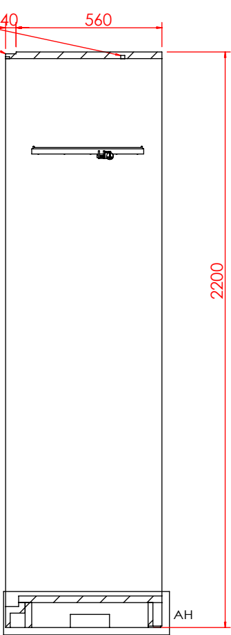
剖面 AG-AG
