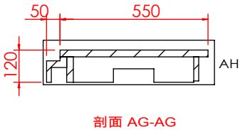
剖面 AG-AG
