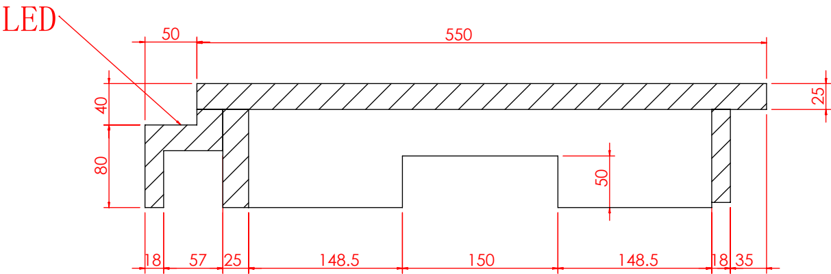
局部视图 AH 比例 1:5
