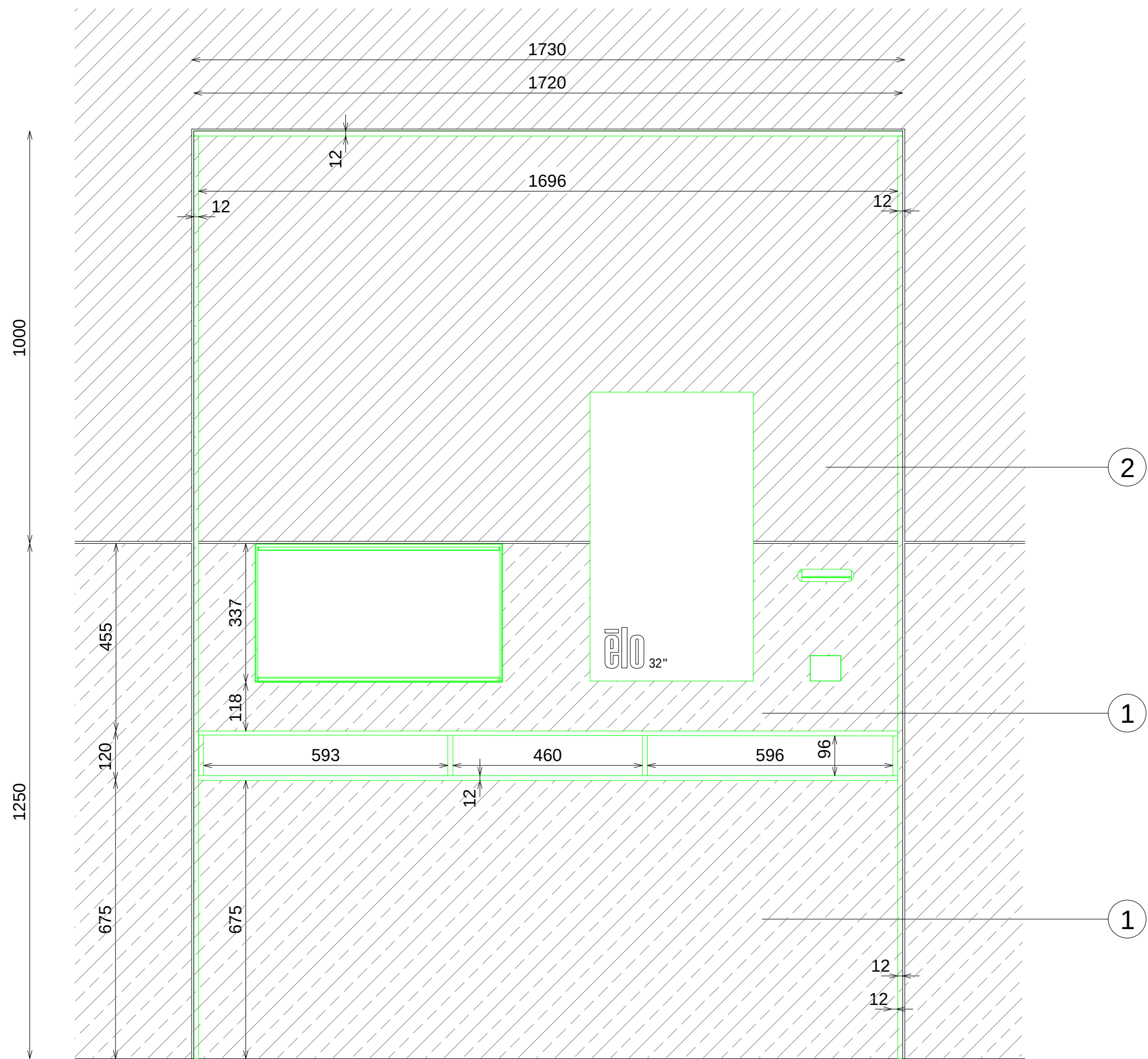
ALZADO FRONTAL
