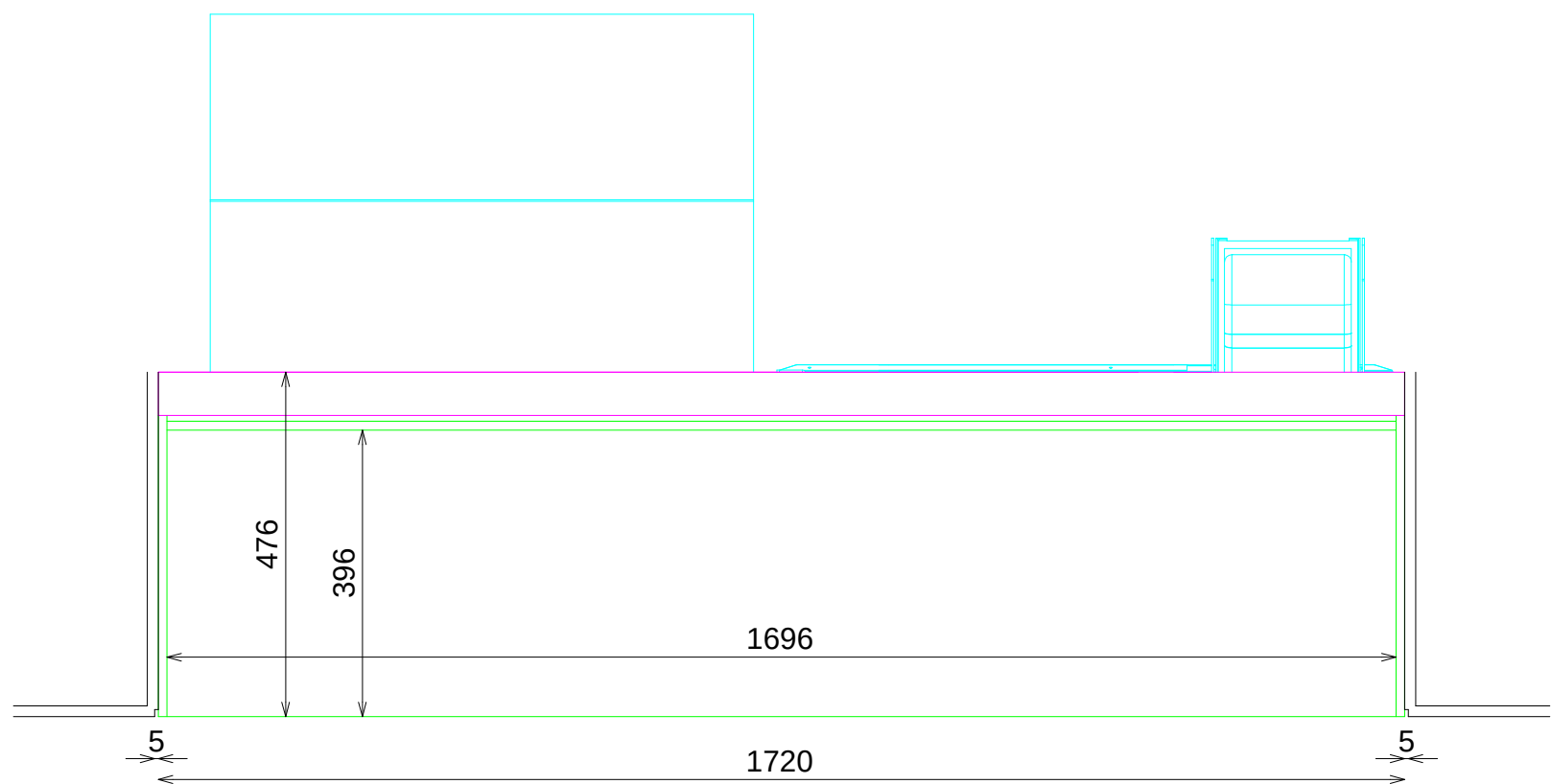
PLANTA
