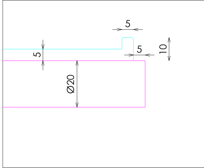
DETALLE B
