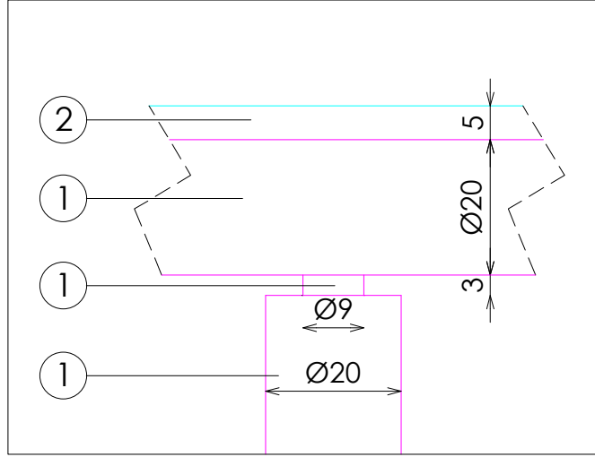
DETALLE A
