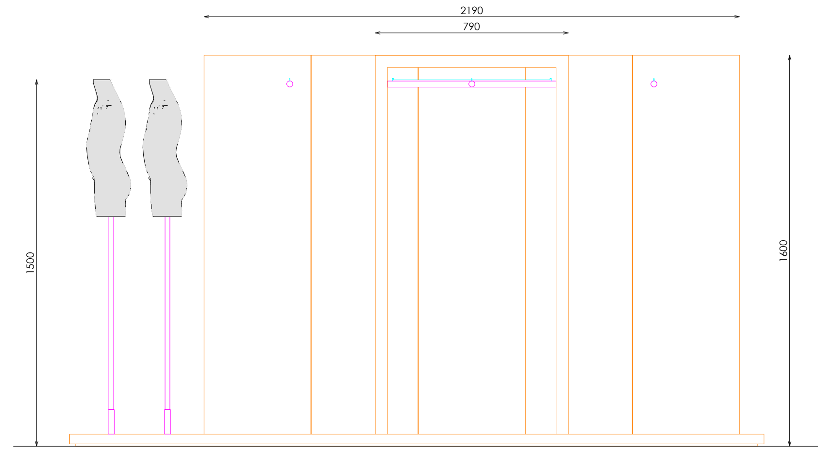
ALZADO FRONTAL
