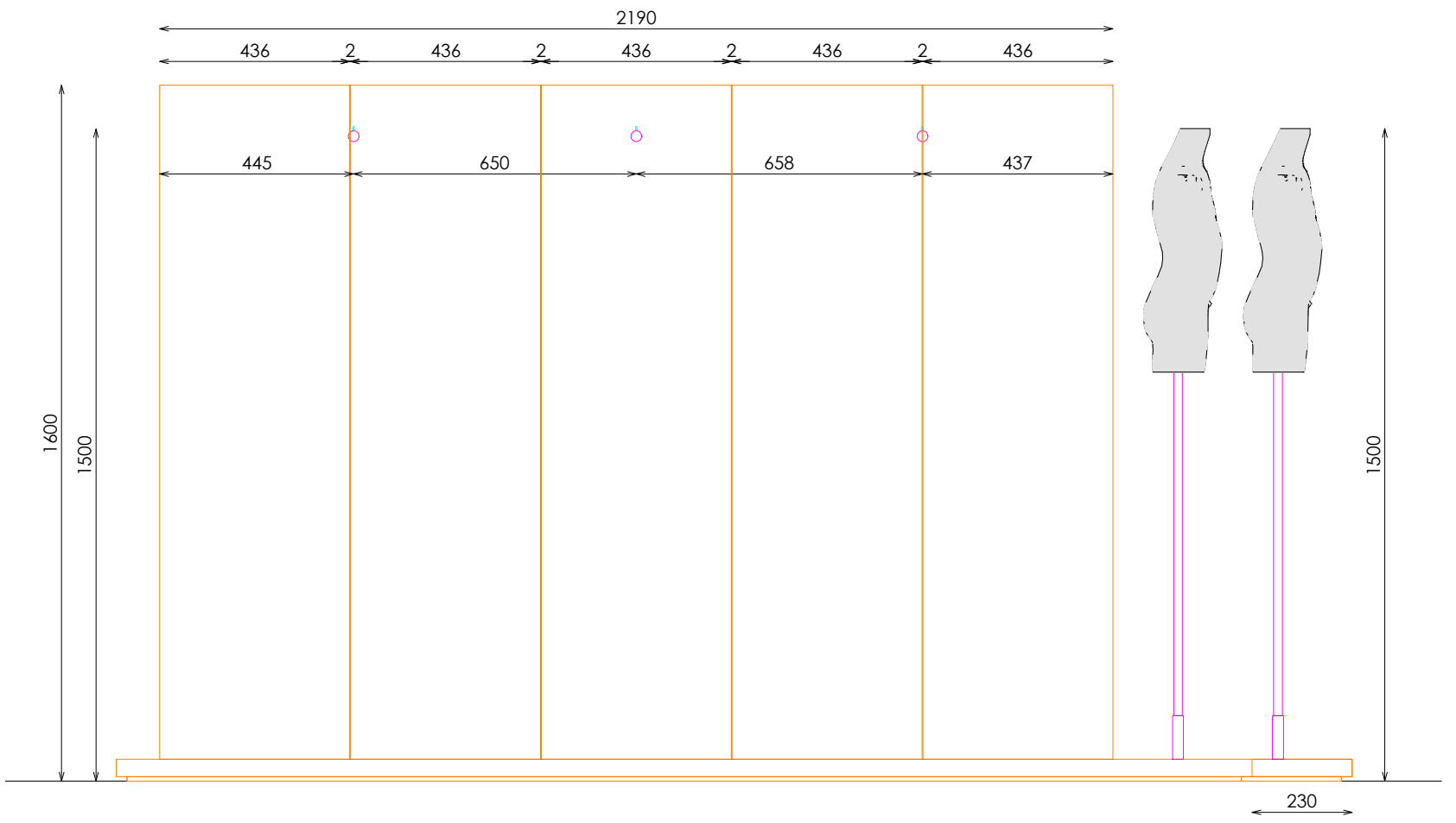
ALZADO POSTERIOR
