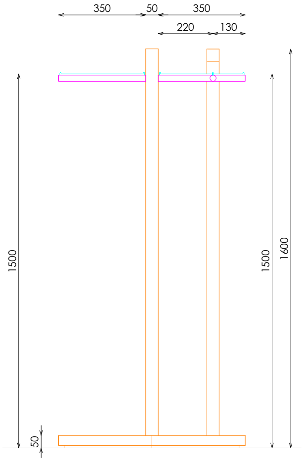
ALZADO LATERAL
