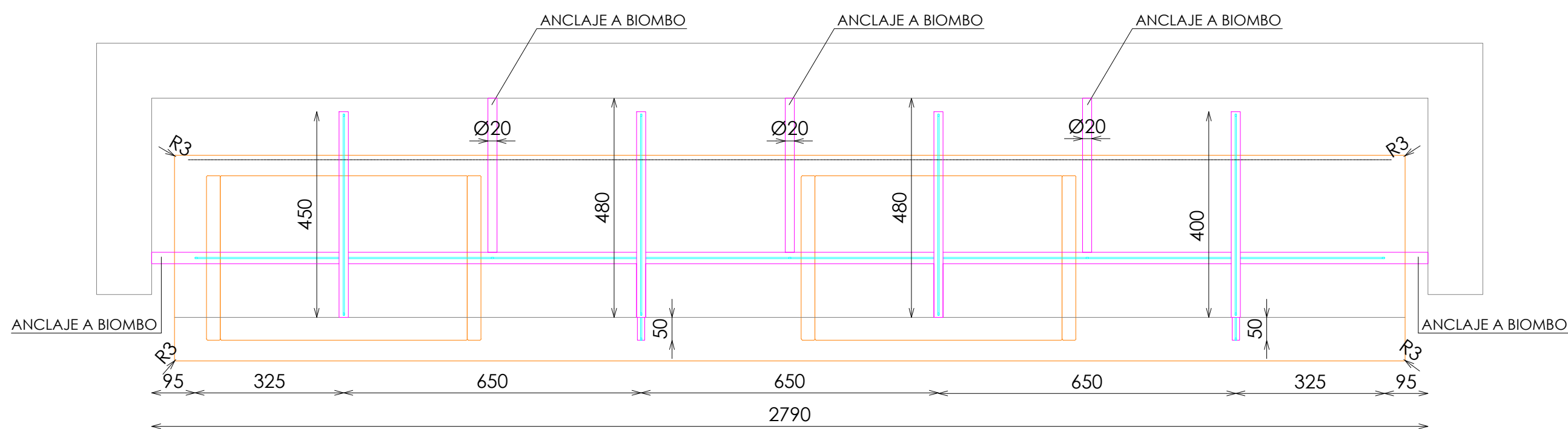
PLANTA
