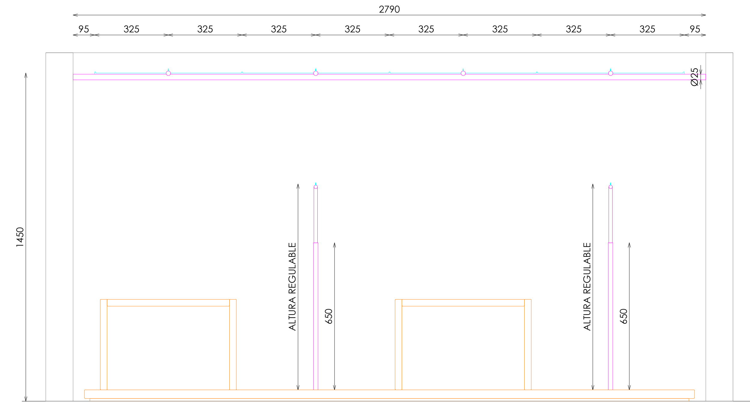
ALZADO FRONTAL
