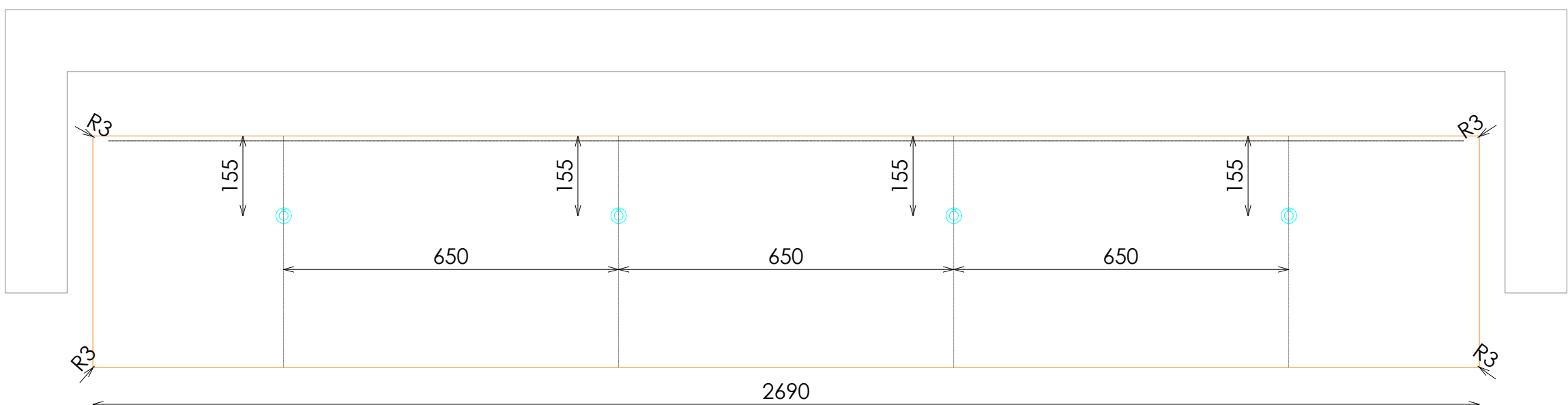
PLANTA TARIMA
