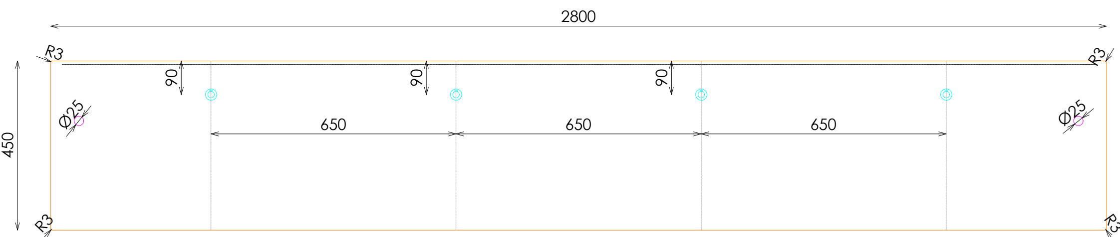
PLANTA TARIMA
