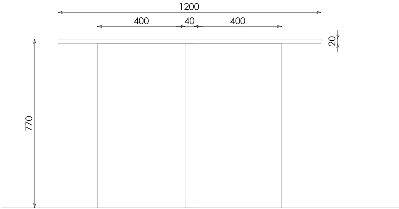
ALZADO LATERAL
