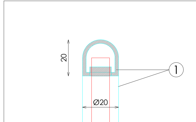
DETALLE SOPORTE PERCHA
