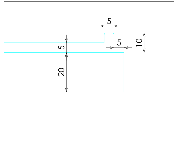
DETALLE B
