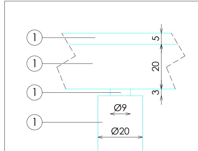
DETALLE A
