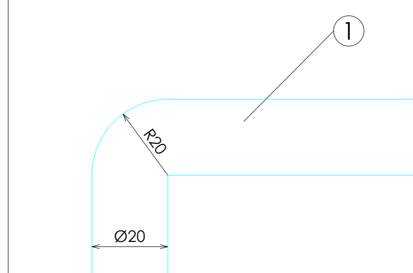
DETALLE SOPORTE PERCHA
