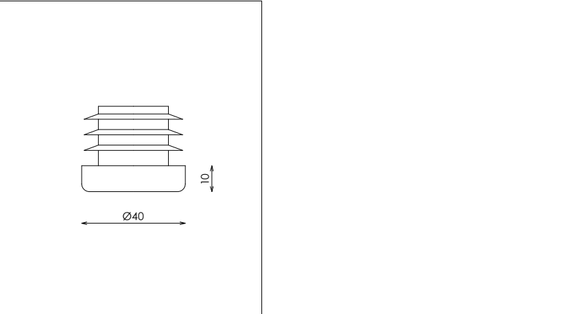
DET. CONTERAS
