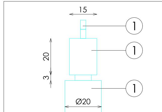
DETALLE C
