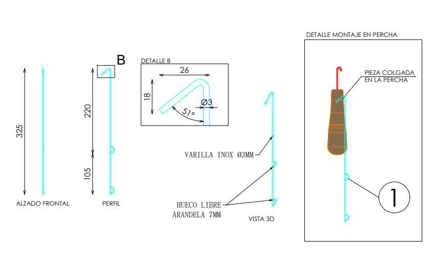
SILUETA PERCHAS (1 UD)
