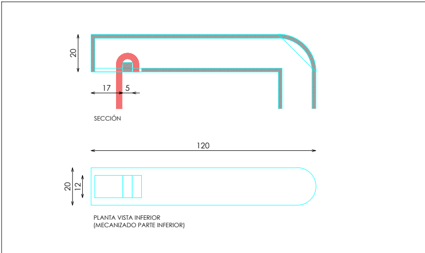
DETALLE SOPORTE PERCHA
