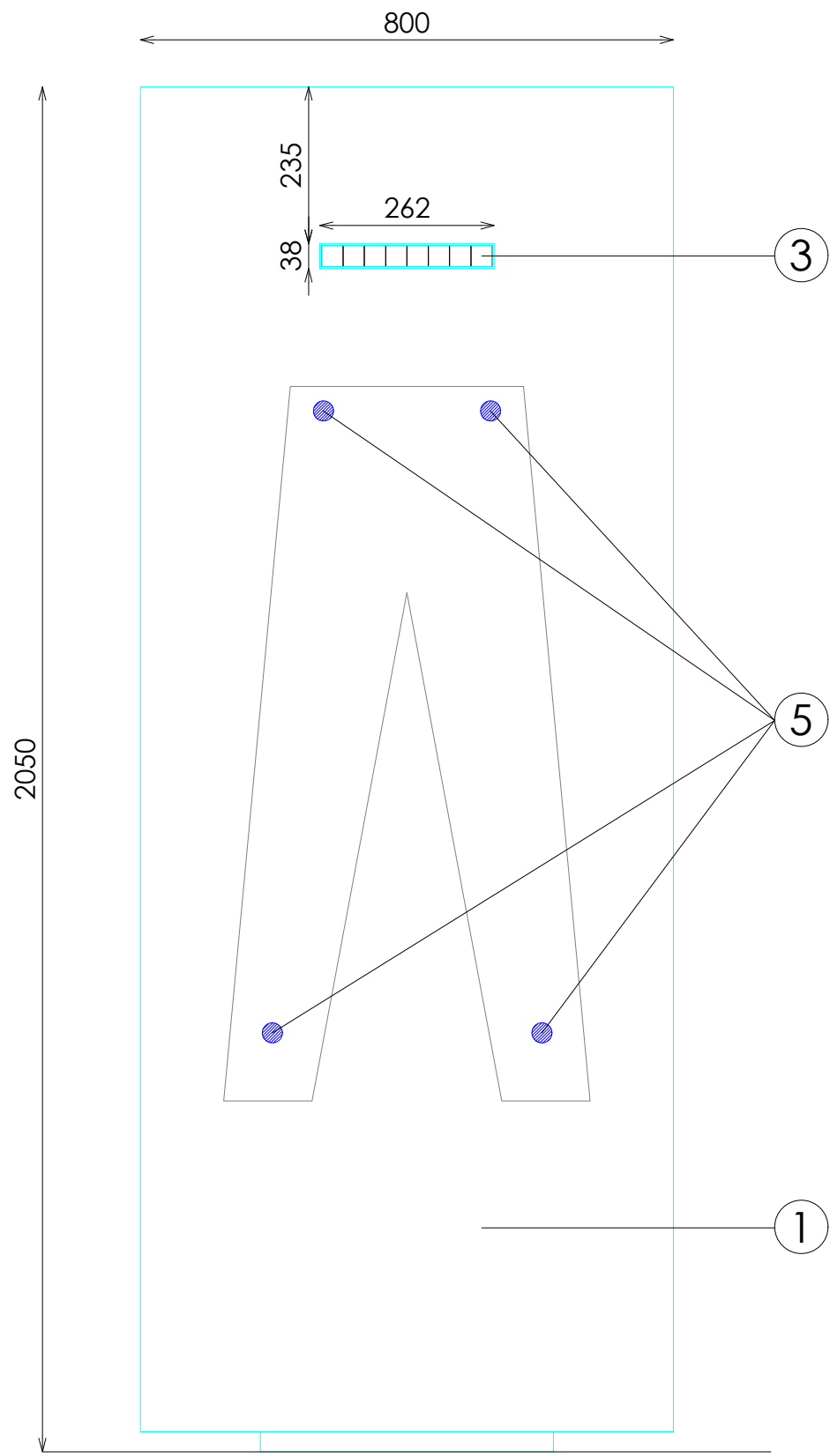
ALZADO
