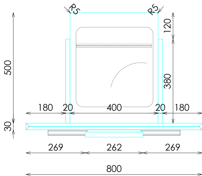
ALZADO
