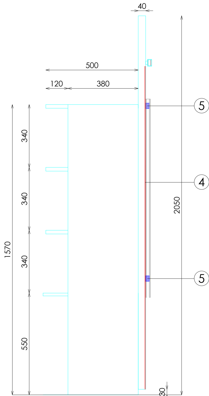
PERFIL
