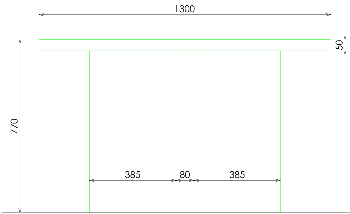
ALZADO LATERAL
