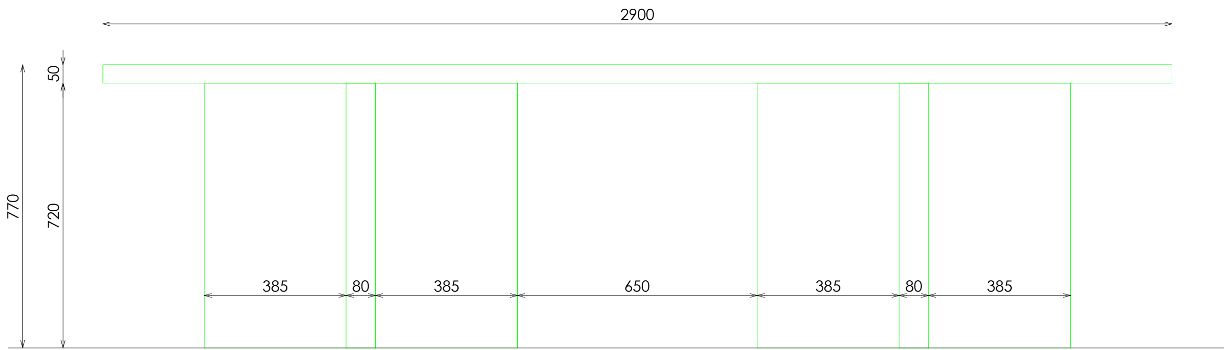
ALZADO FRONTAL
