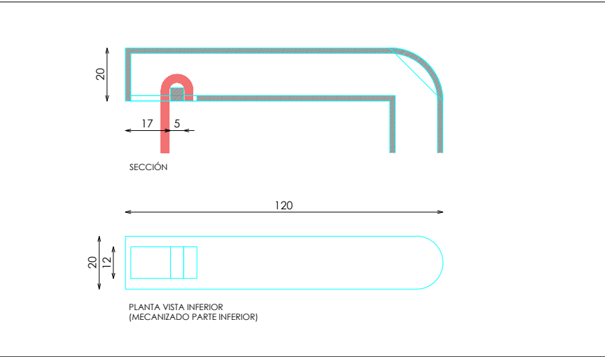
DETALLE TUBO SUPERIOR
