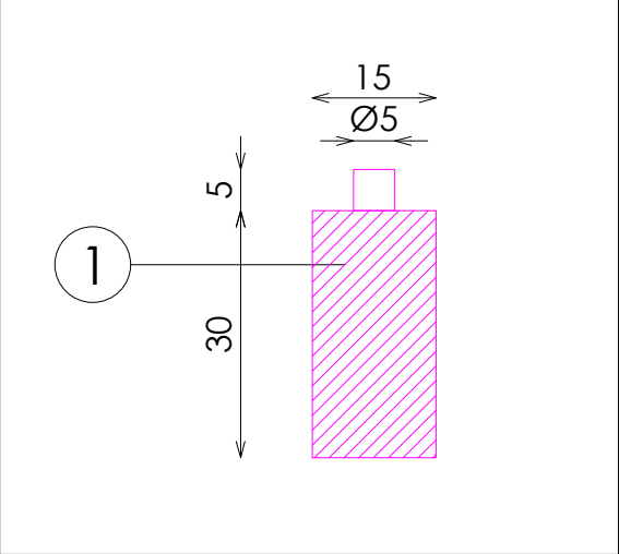
DETALLE BARRA
