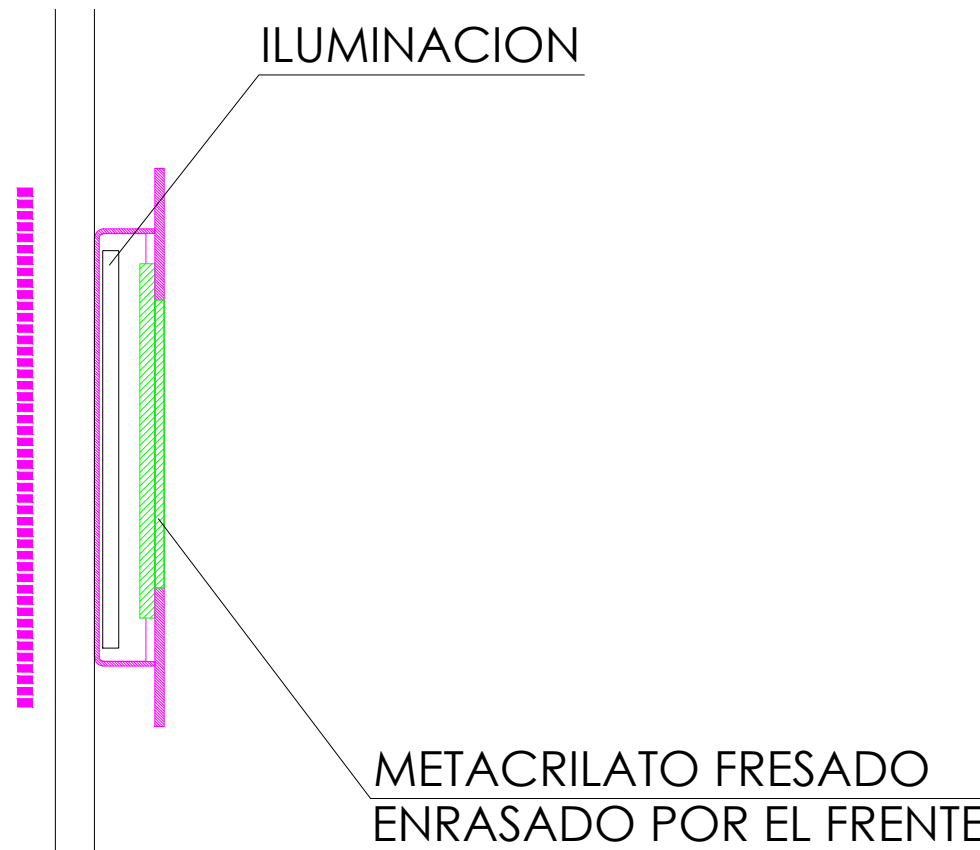
SECCIÓN
