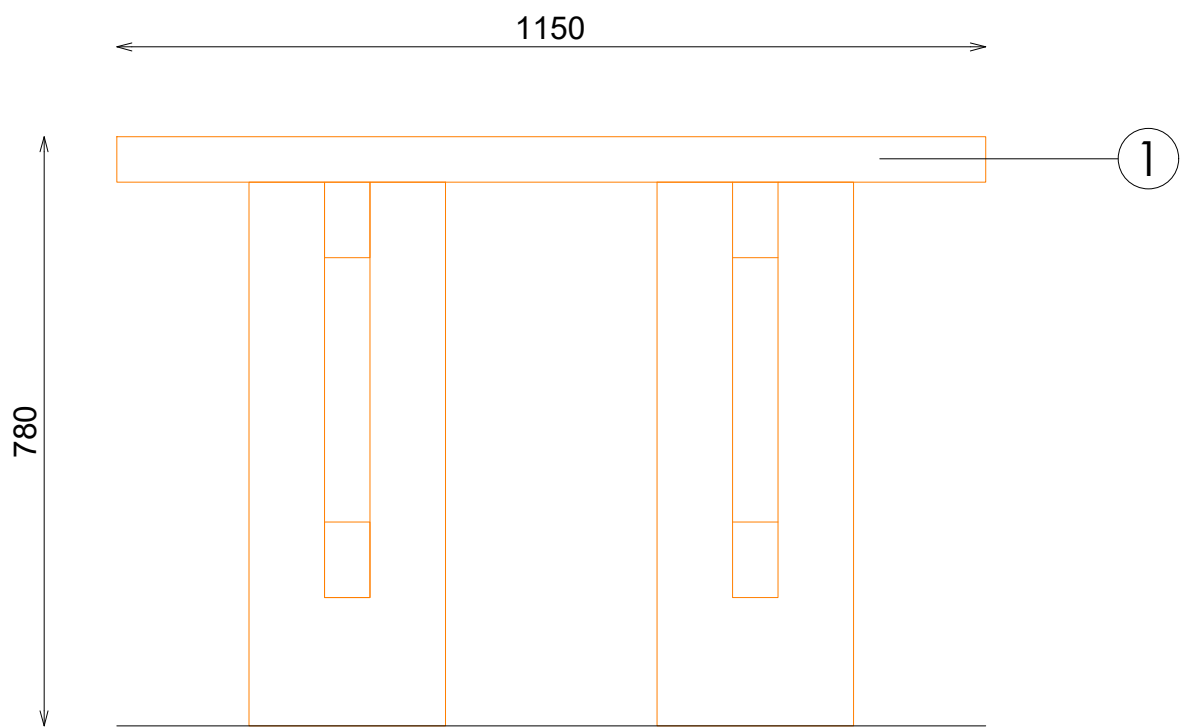
ALZADO LATERAL
