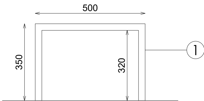
ALZADO
