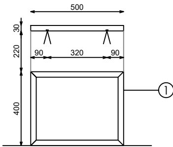
SECCION
