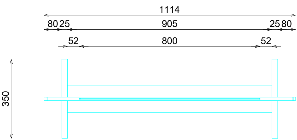
PLANTA
