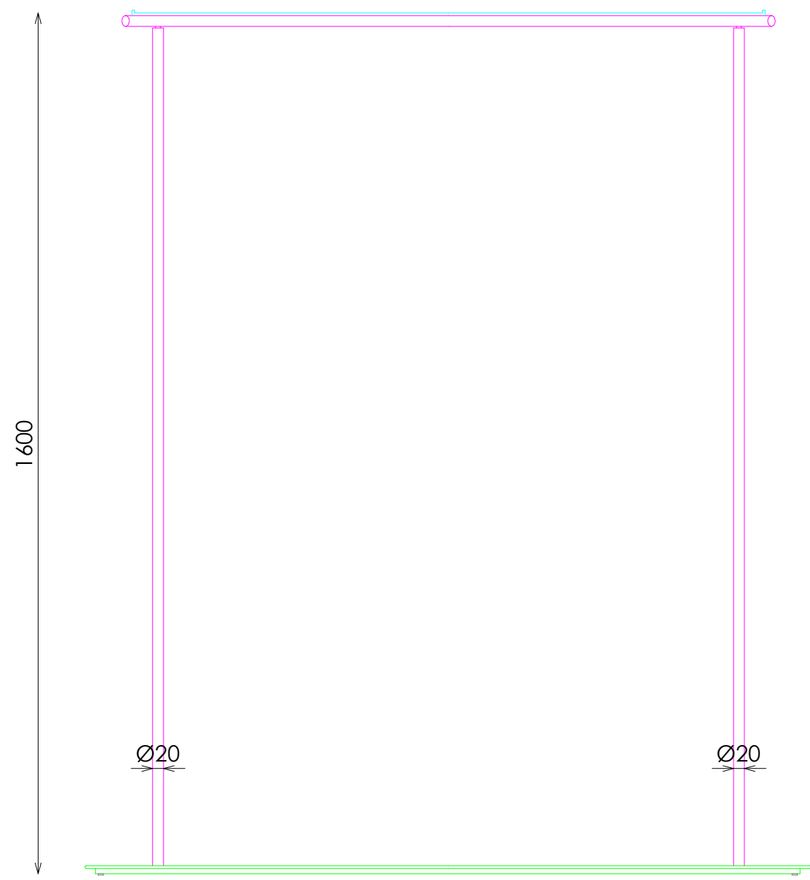
ALZADO
