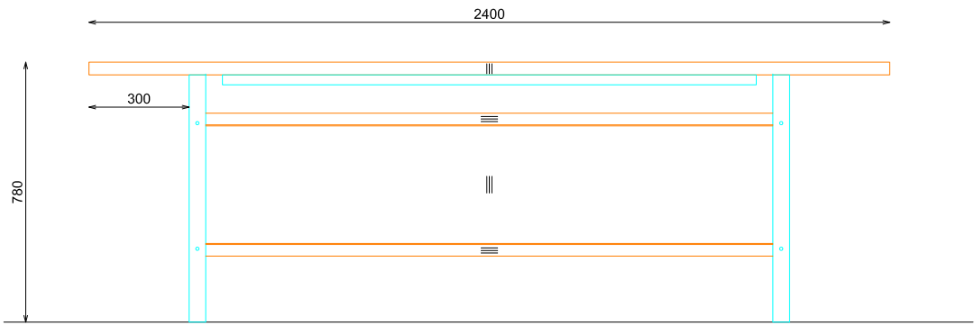
ALZADO FRONTAL
