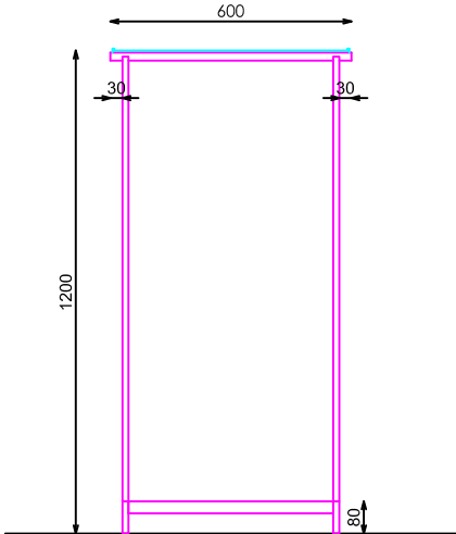
ALZADO
