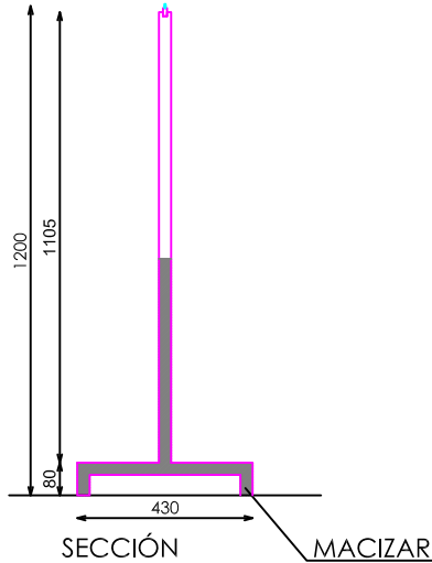
SECCIÓN
