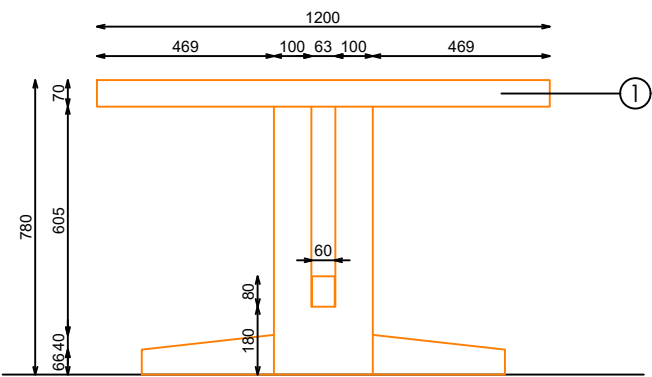
ALZADO LATERAL
