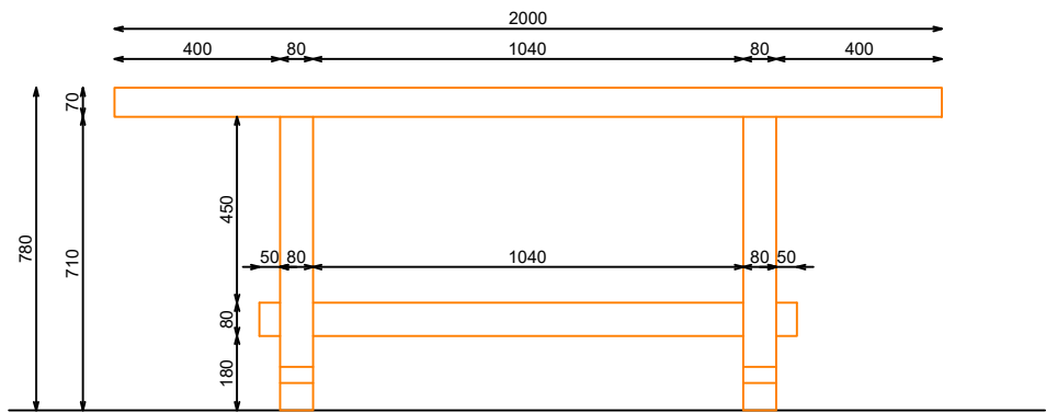
ALZADO FRONTAL
