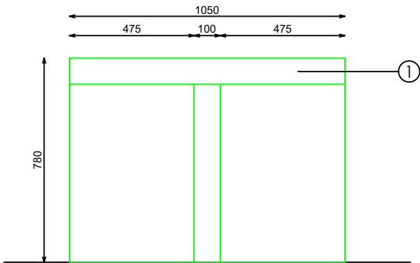
ALZADO LATERAL
