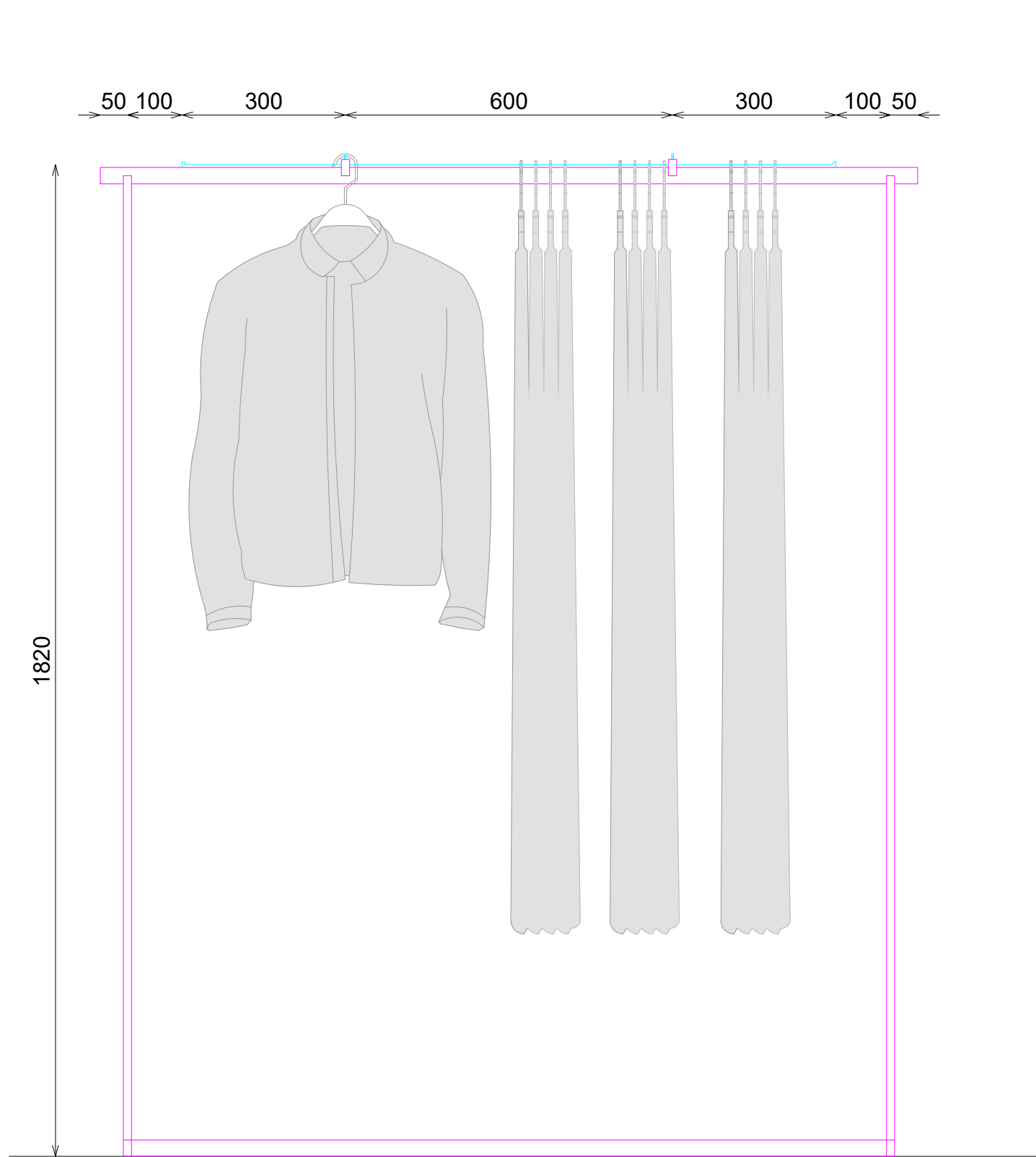
ALZADO
