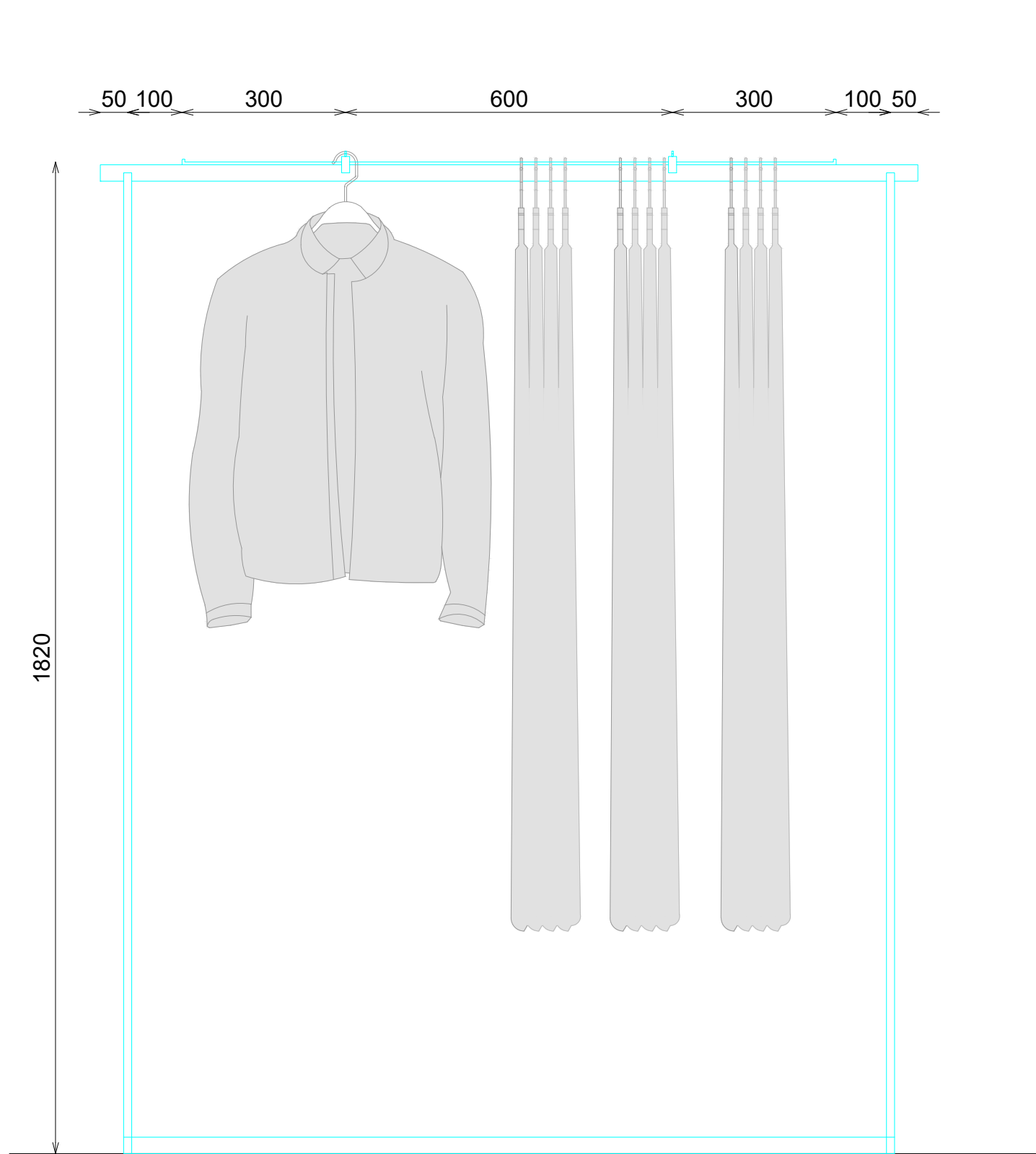
ALZADO
