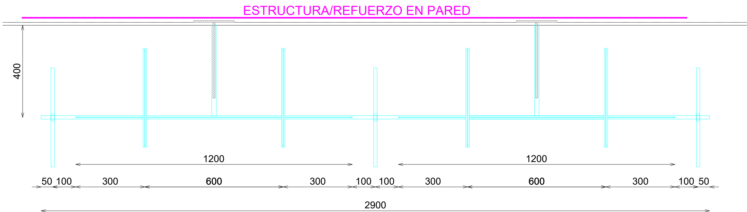
PLANTA
