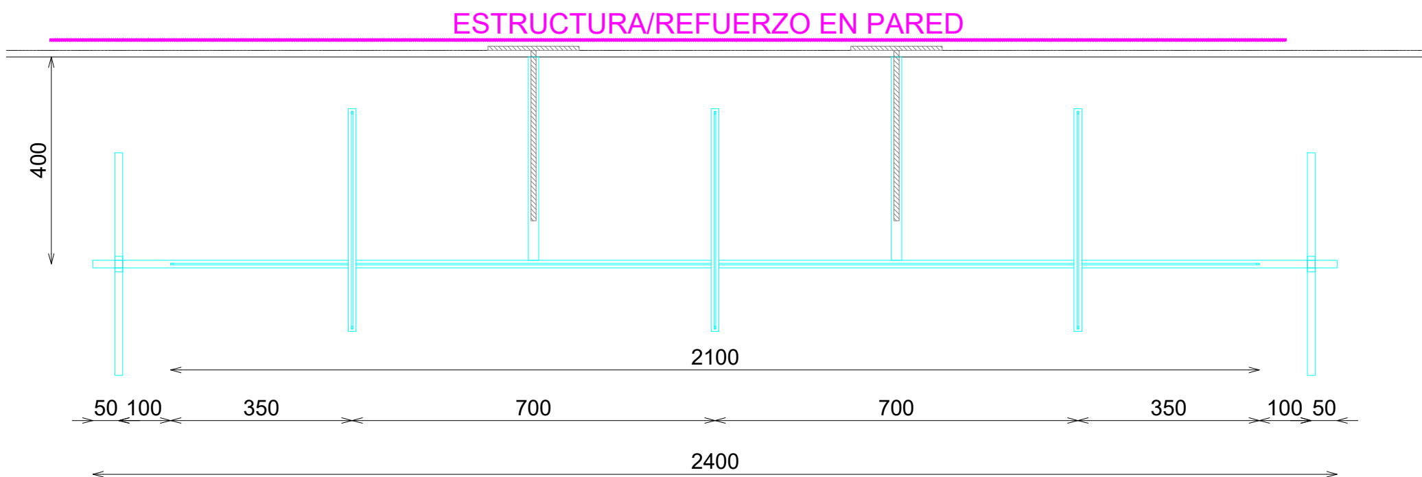
PLANTA
