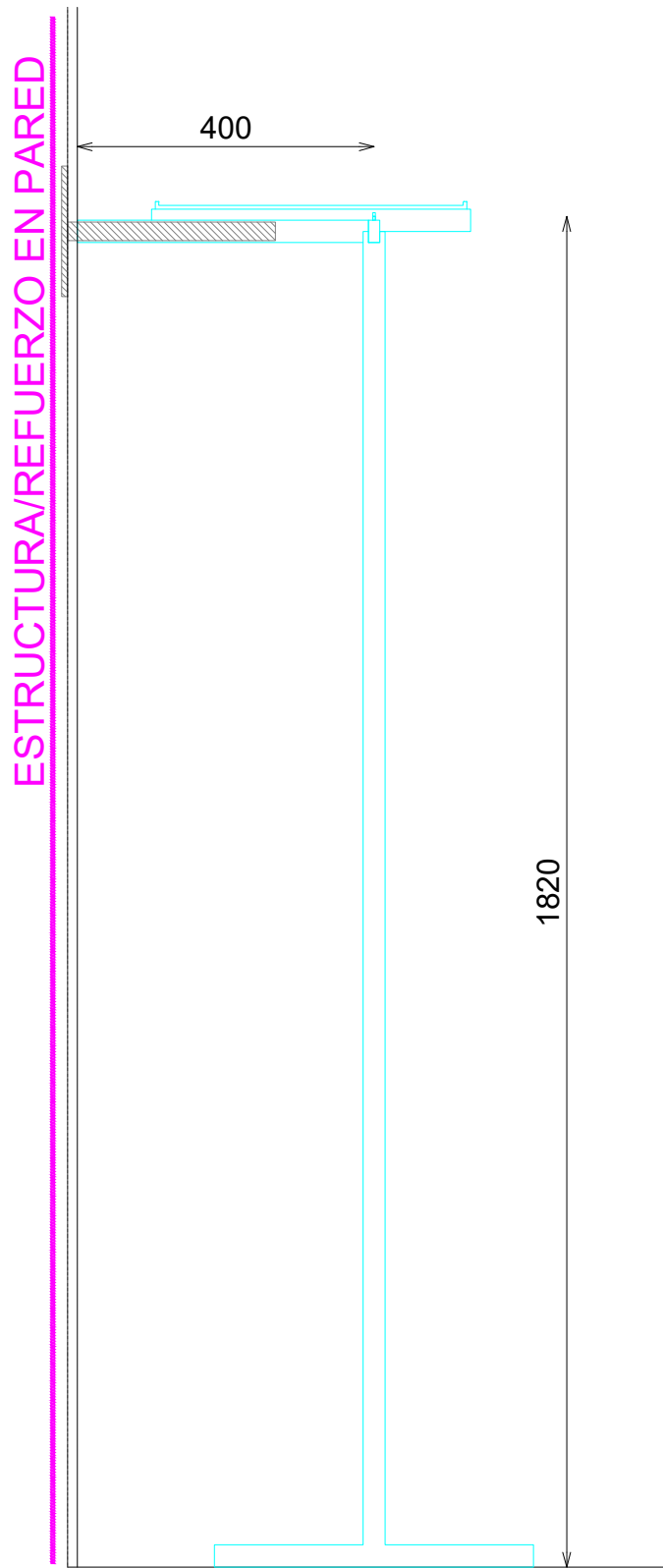
SECCION
