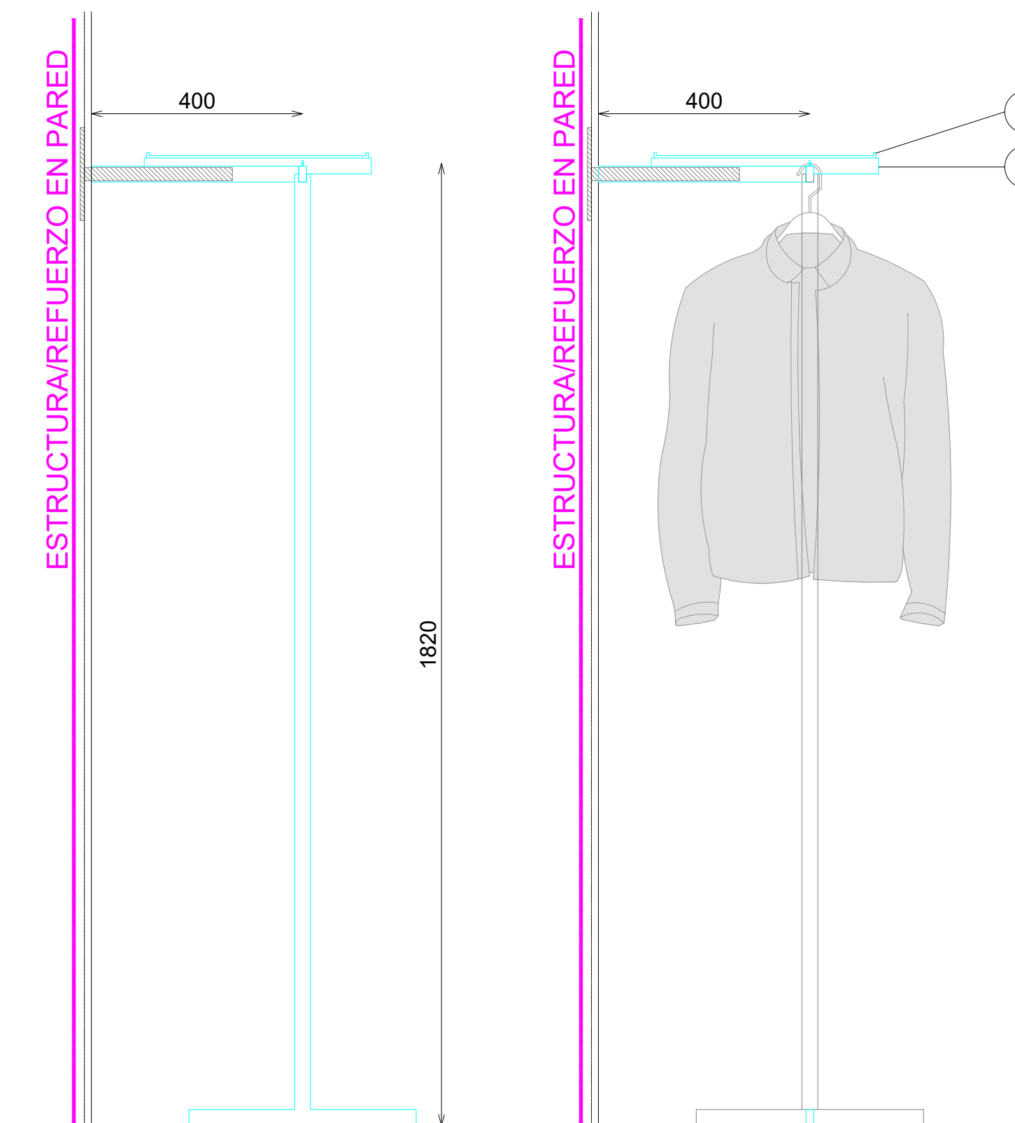
SECCION
