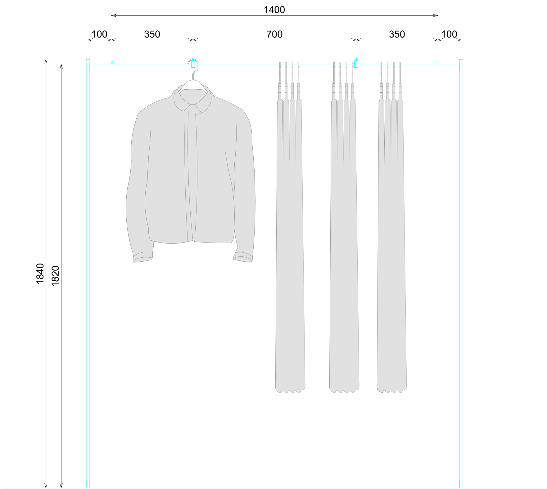
ALZADO SECCIONADO
