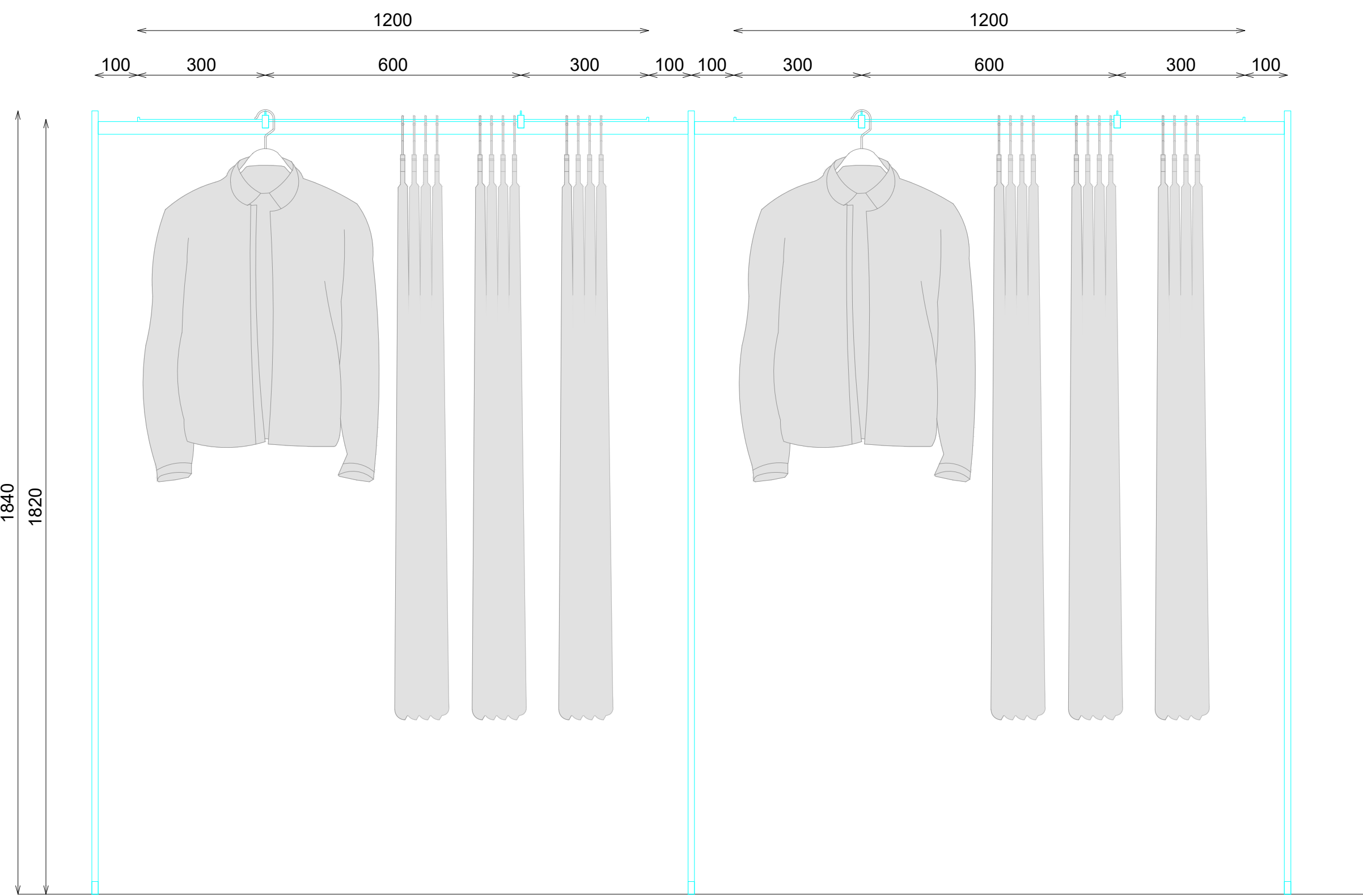
ALZADO SECCIONADO
