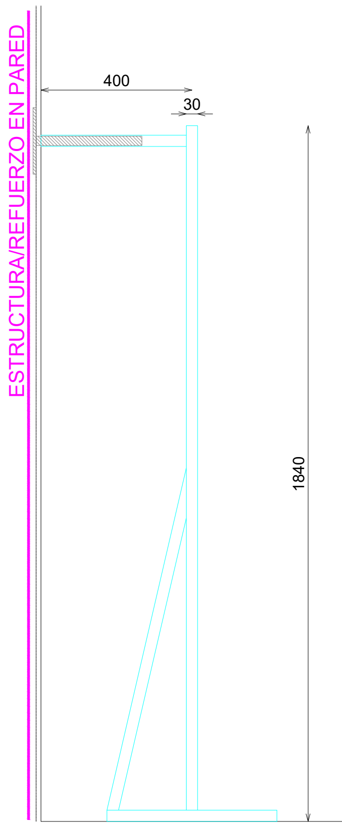
PERFIL
