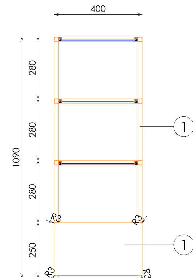
SECCIÓN
