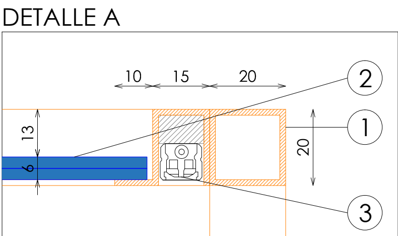
DETALLE A
