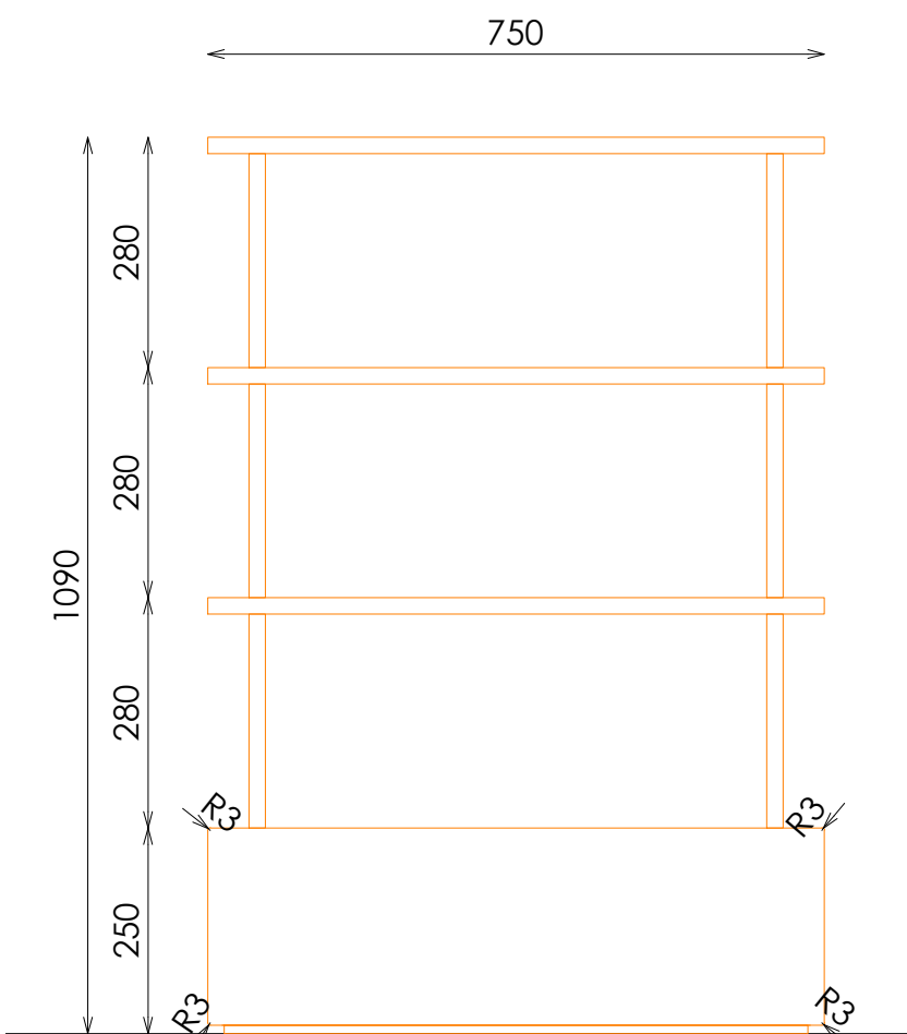
ALZADO
