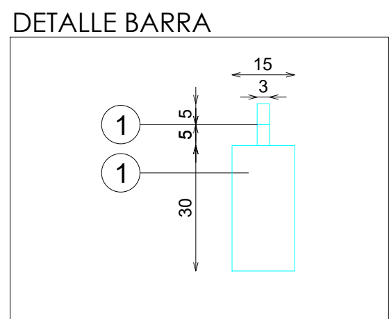
DETALLE BARRA
