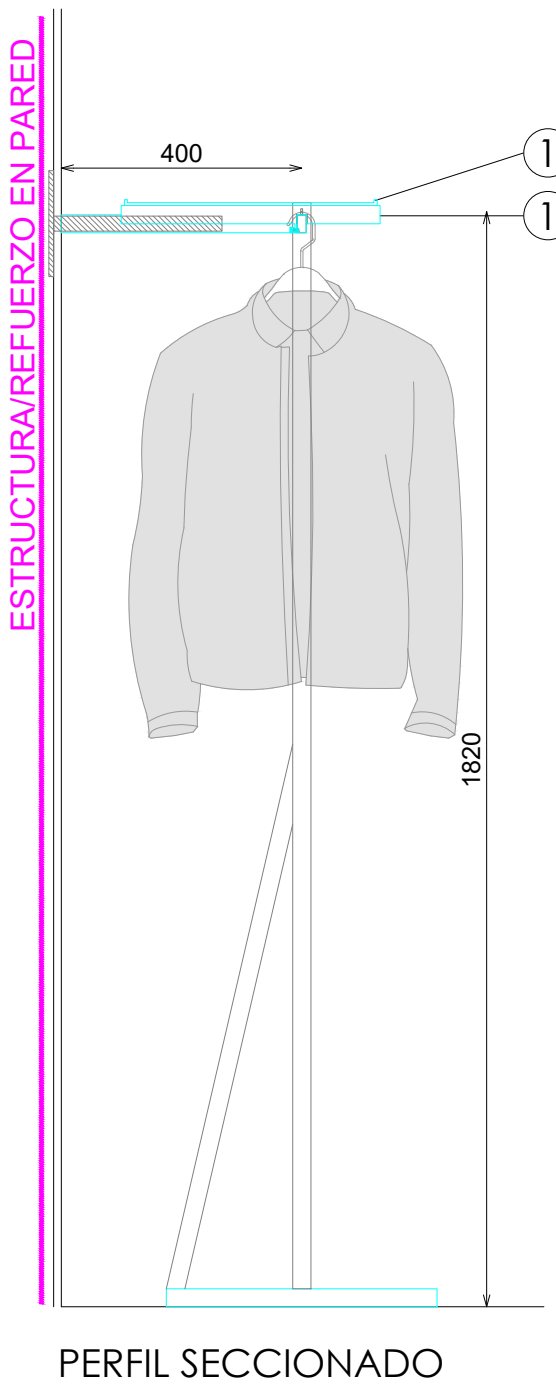
PERFIL SECCIONADO
