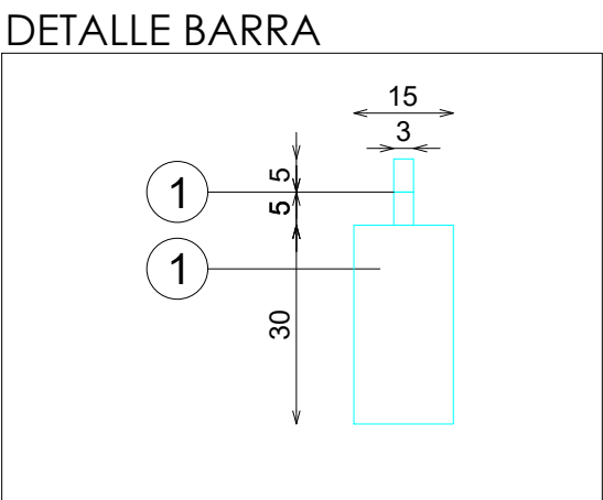
DETALLE BARRA
