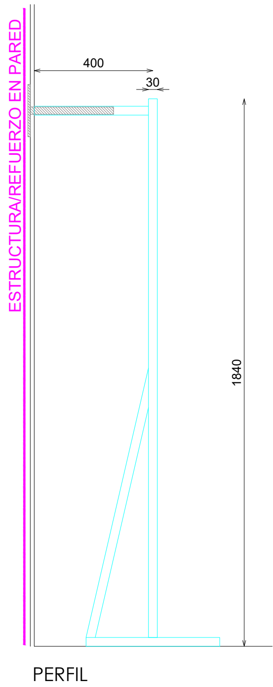
PERFIL
