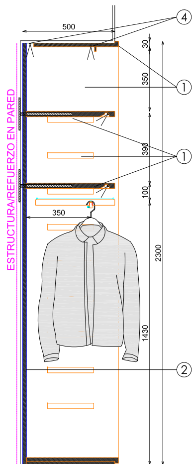
SECCION BARRA BAJA
