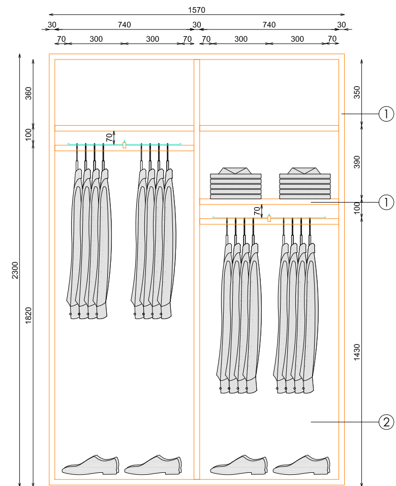
ALZADO
