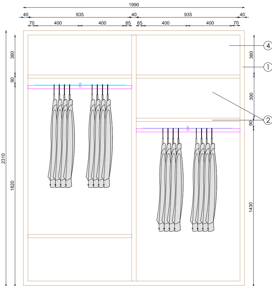
ALZADO
