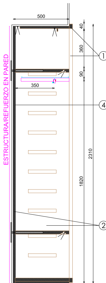
SECCION BARRA ALTA
