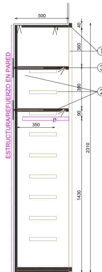
SECCION BARRA BAJA
