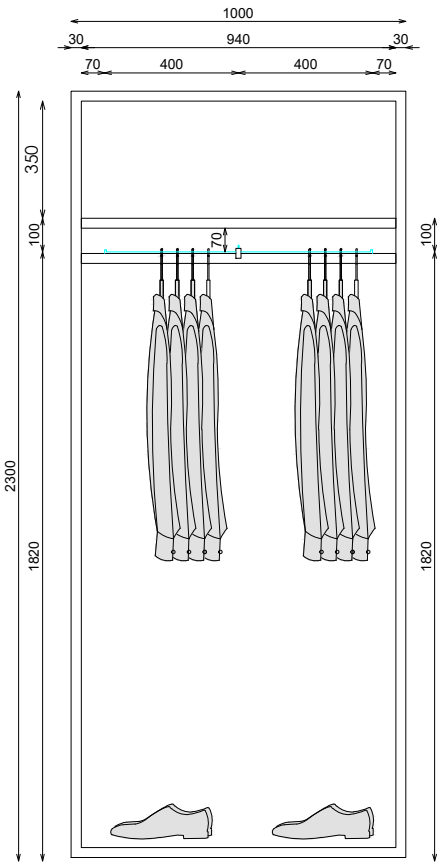
ALZADO
