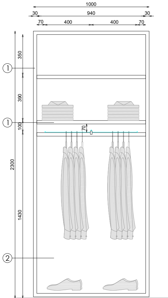
ALZADO
