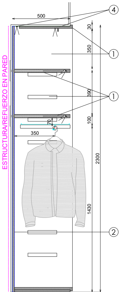
SECCION
