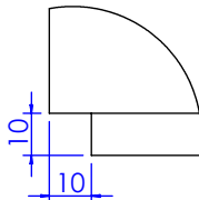
局部视图 AM 比例 1:2
