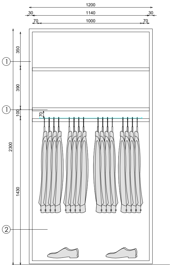
ALZADO
