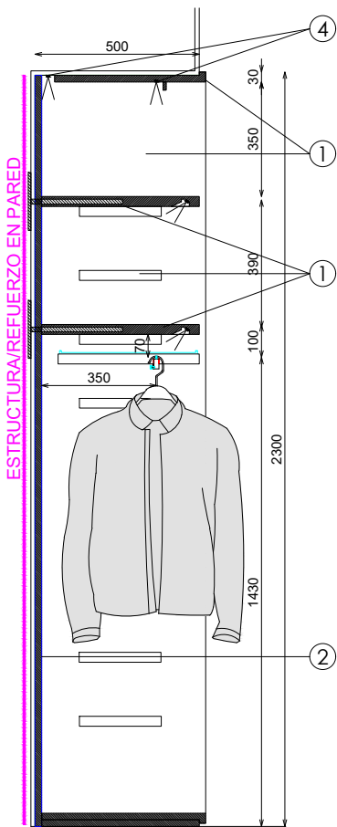
SECCION
