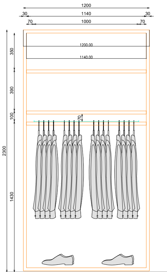
ALZADO
