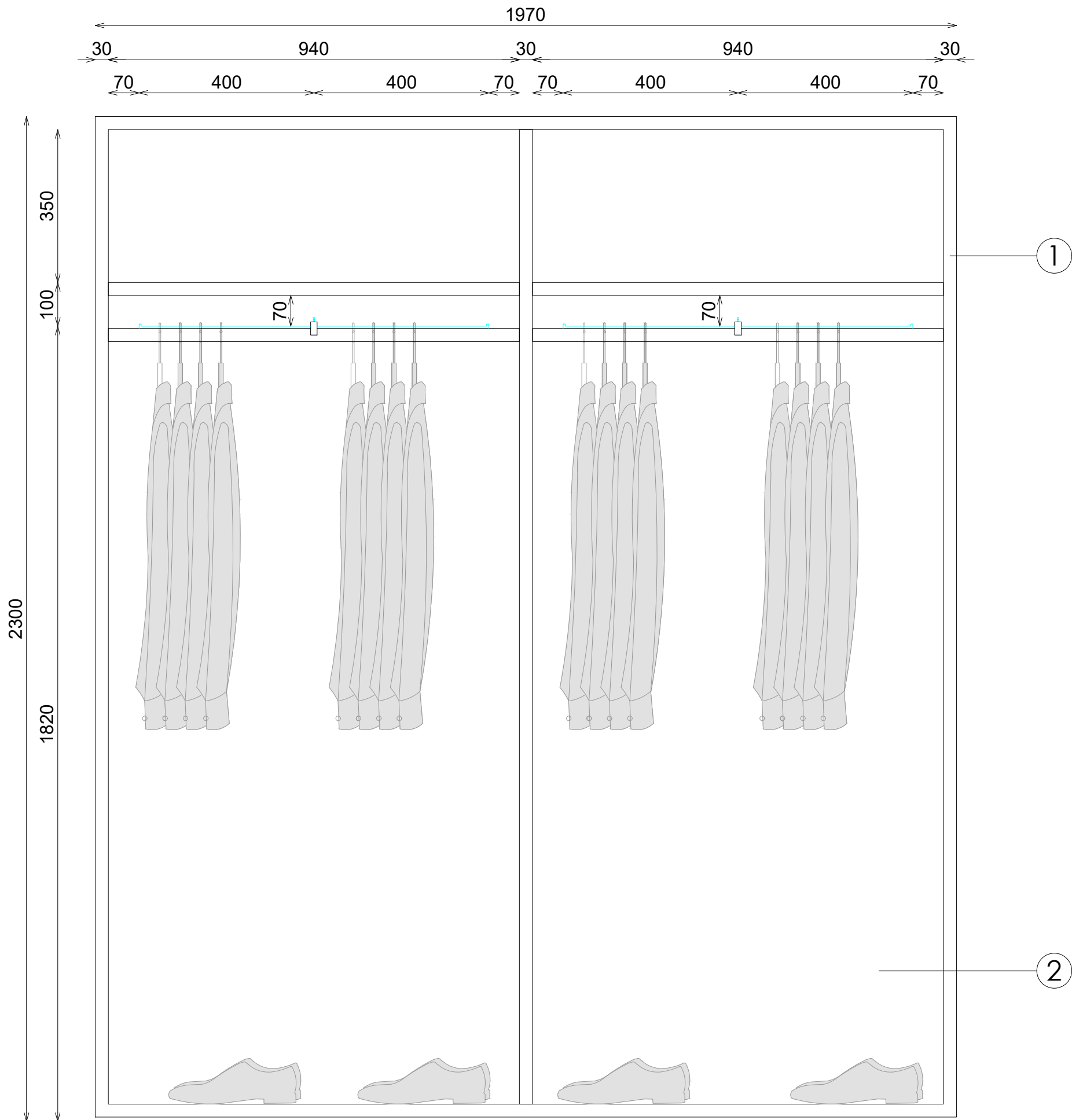
ALZADO
