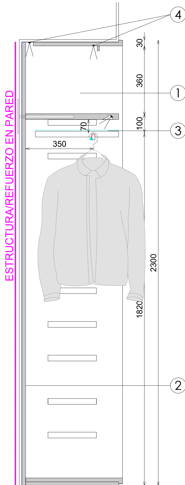
SECCION
