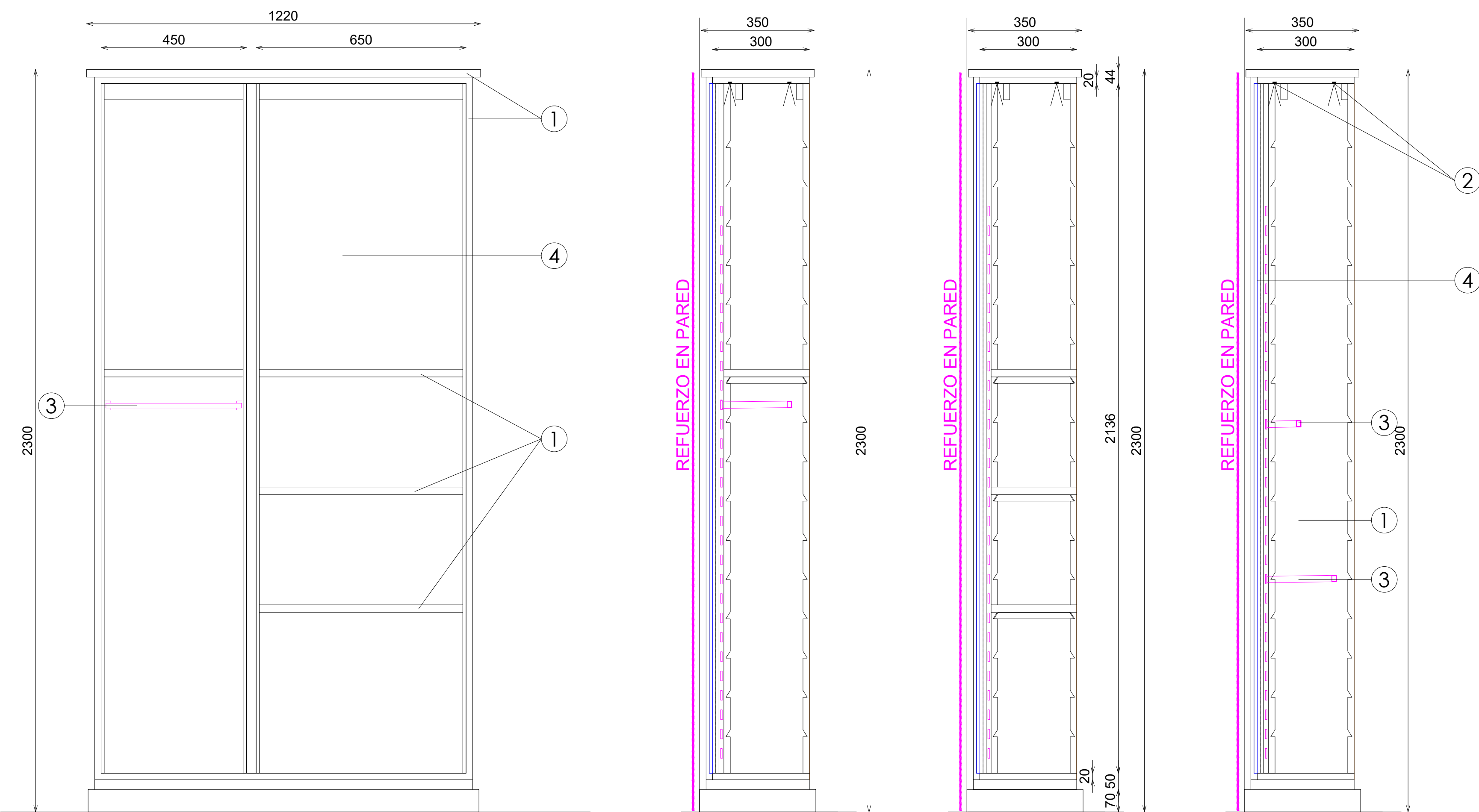
ALZADO FRONTAL ABIERTO
