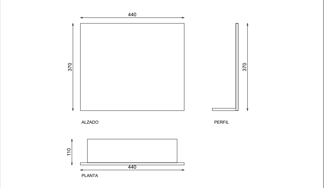
DETALLE CAJON CINTURONES (MODULO 45)
