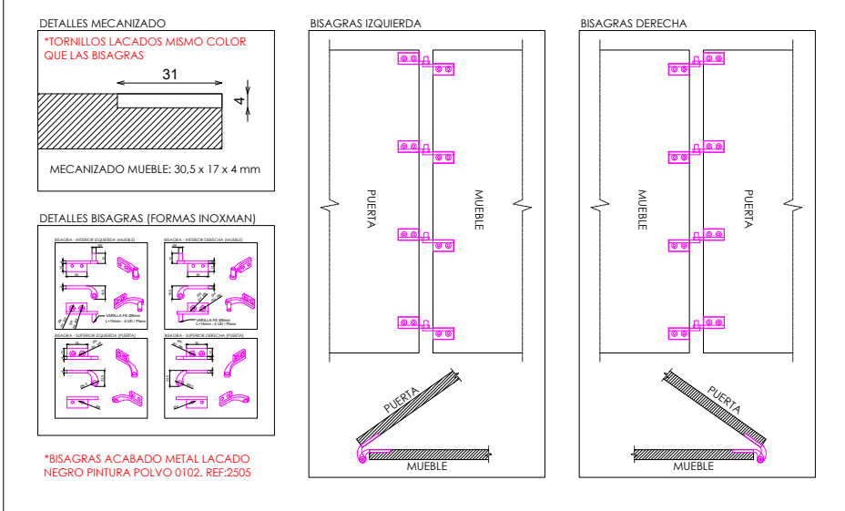
DETALLE BISAGRAS. FORMAS INOXMAN
