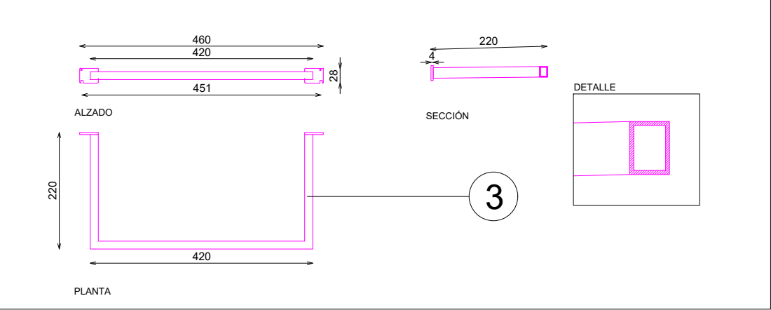
DETALLE BARRA 220 (MODULO 45)
