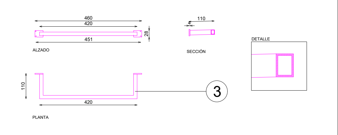
DETALLE BARRA 110 (MODULO 45)
