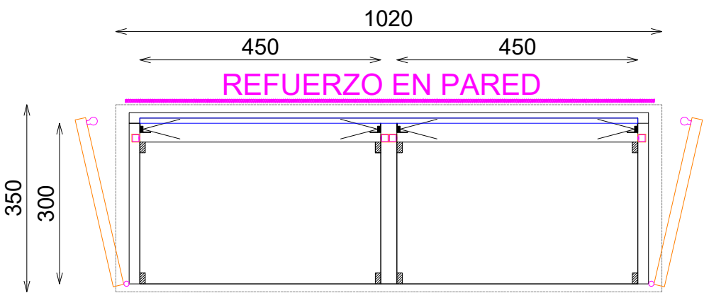
PLANTA SECCIONADA BALDAS
