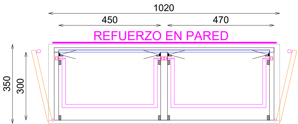
PLANTA SECCIONADA DOTACION BARRAS/PINCHOS
