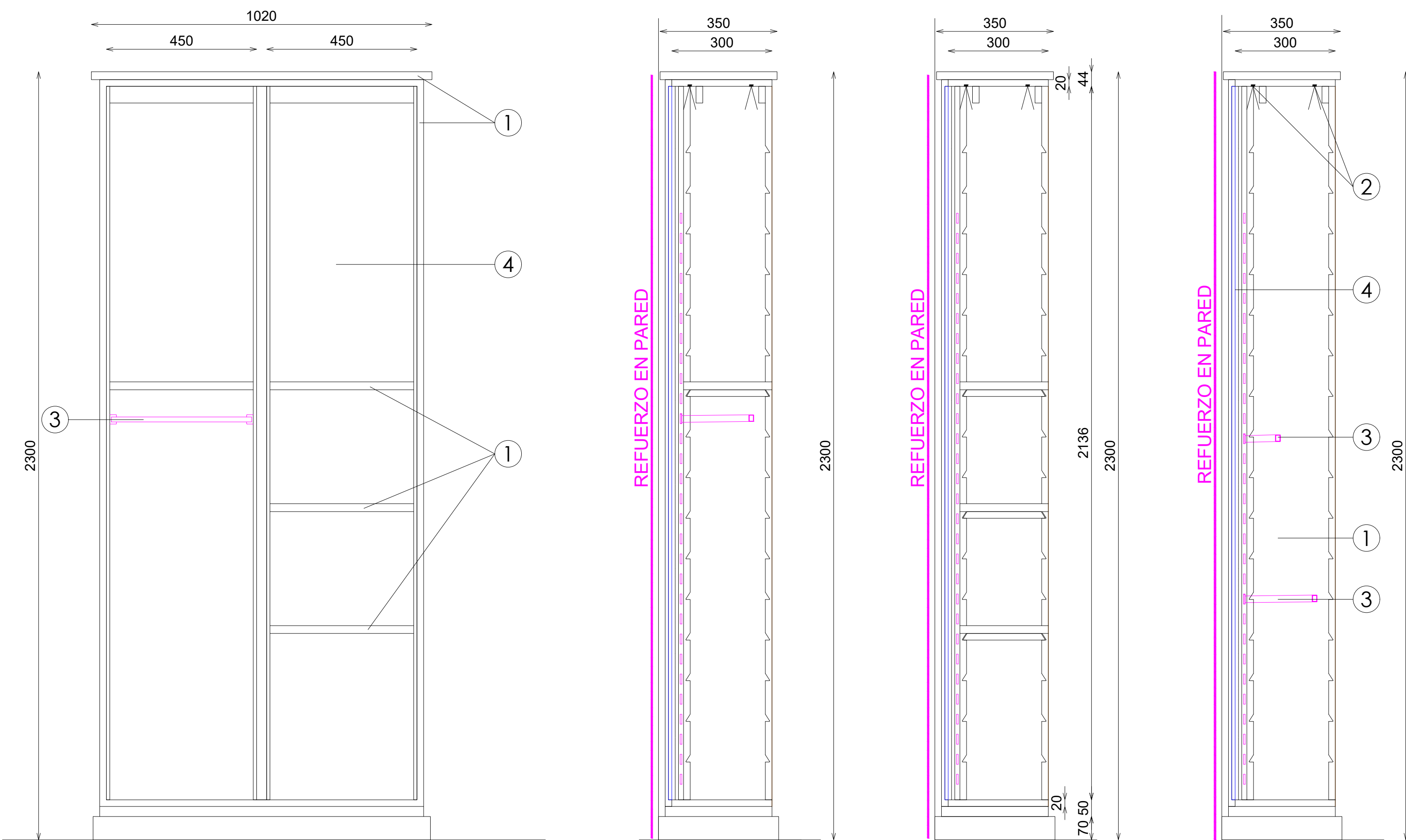
ALZADO FRONTAL ABIERTO
