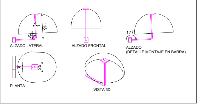
DETALLE CAJON CINTURONES (MODULO 45)
